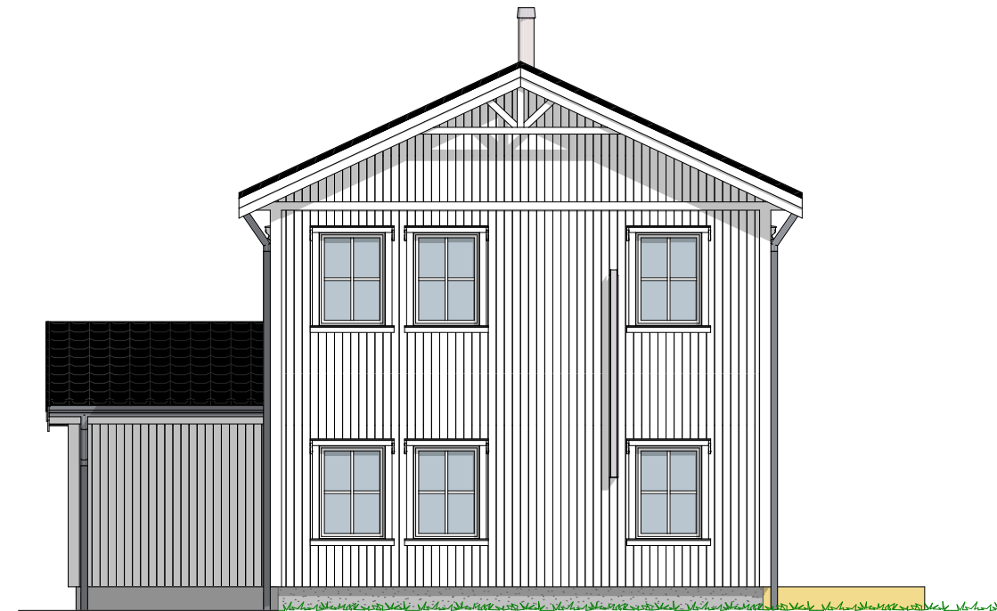
1:100 Fasade Vest
