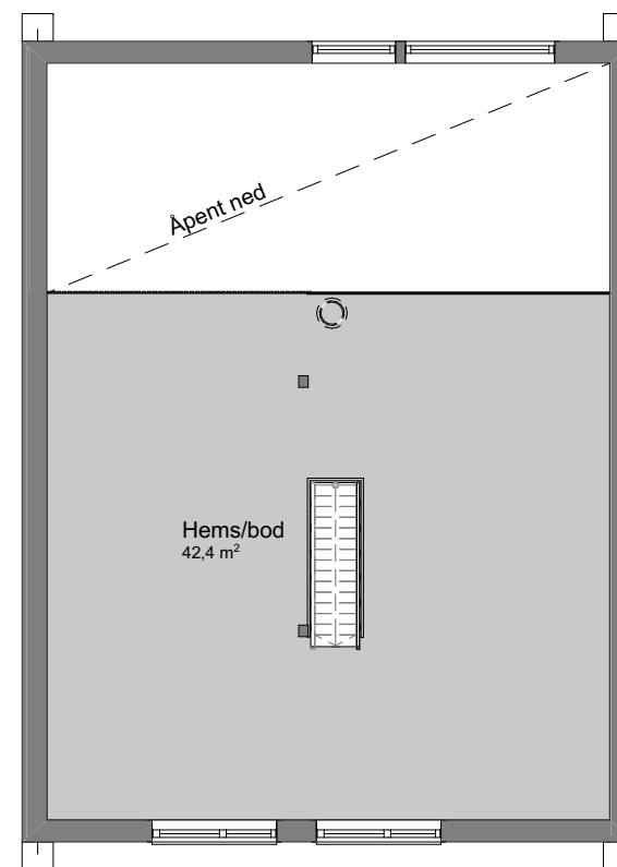
1:100 Hems
