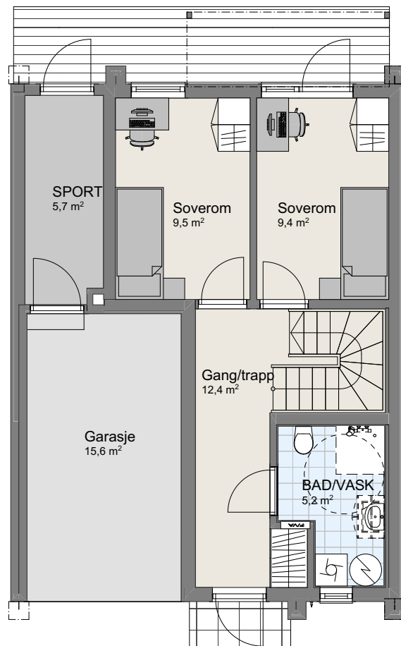
1:100 H. Etasje
