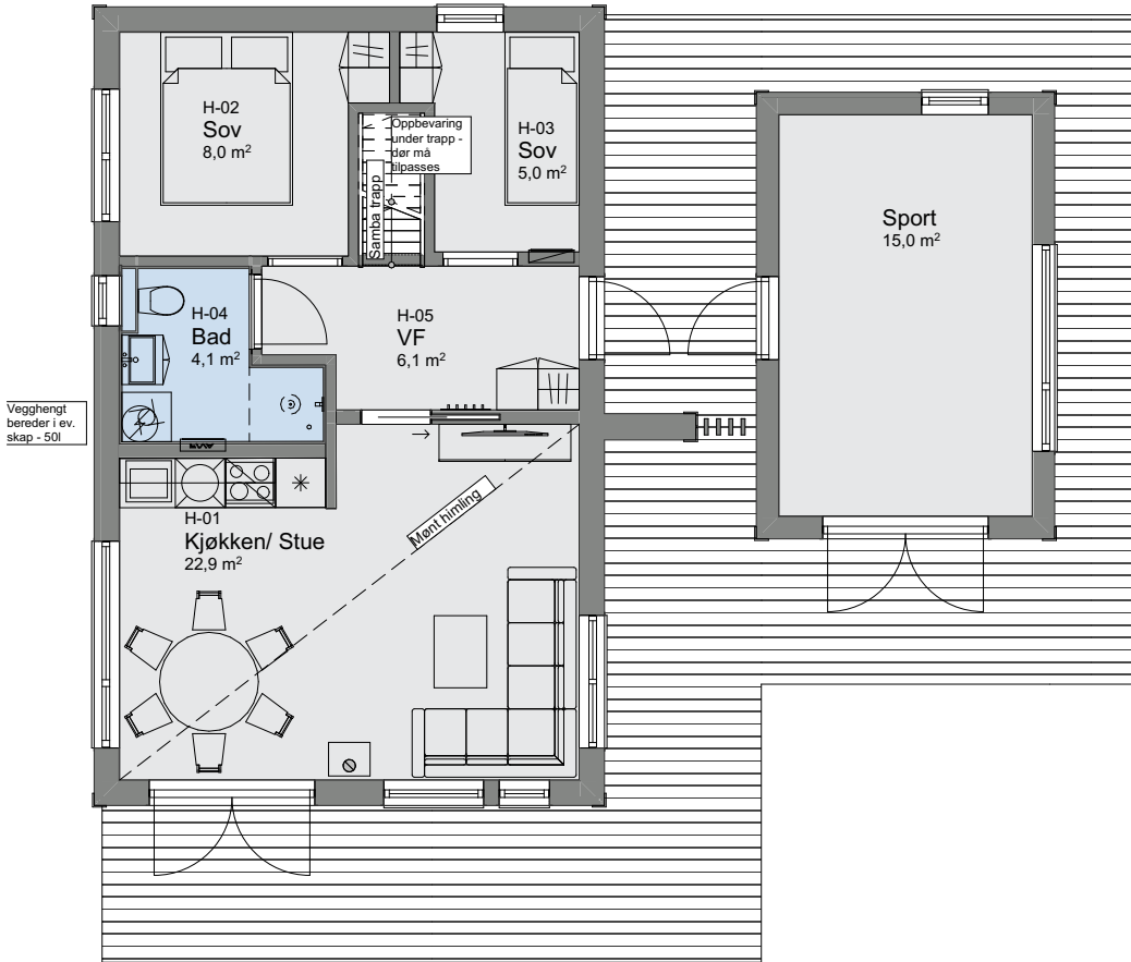
1:100 H. etasje
