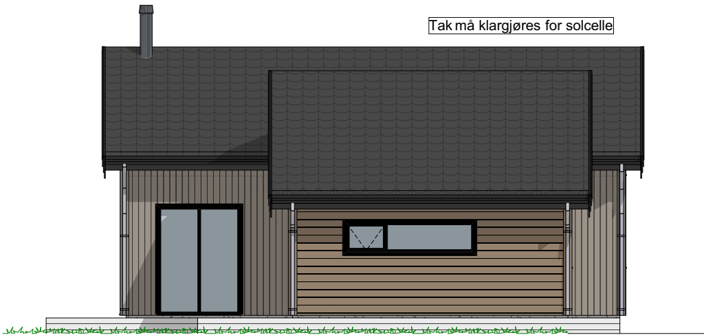
1:100 Fasade SørØst
