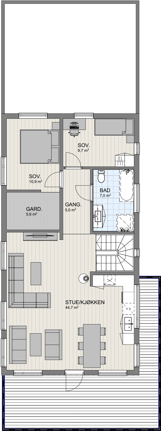
1:100 H. Etasje
