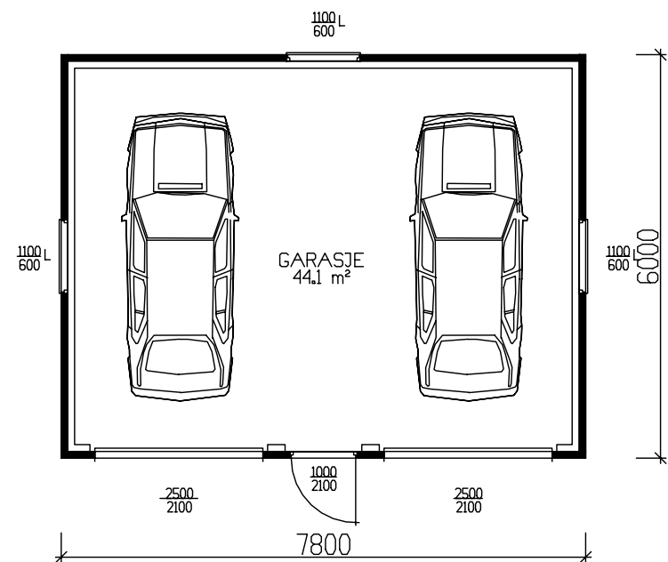
GARASJE 44,1m² BRA
