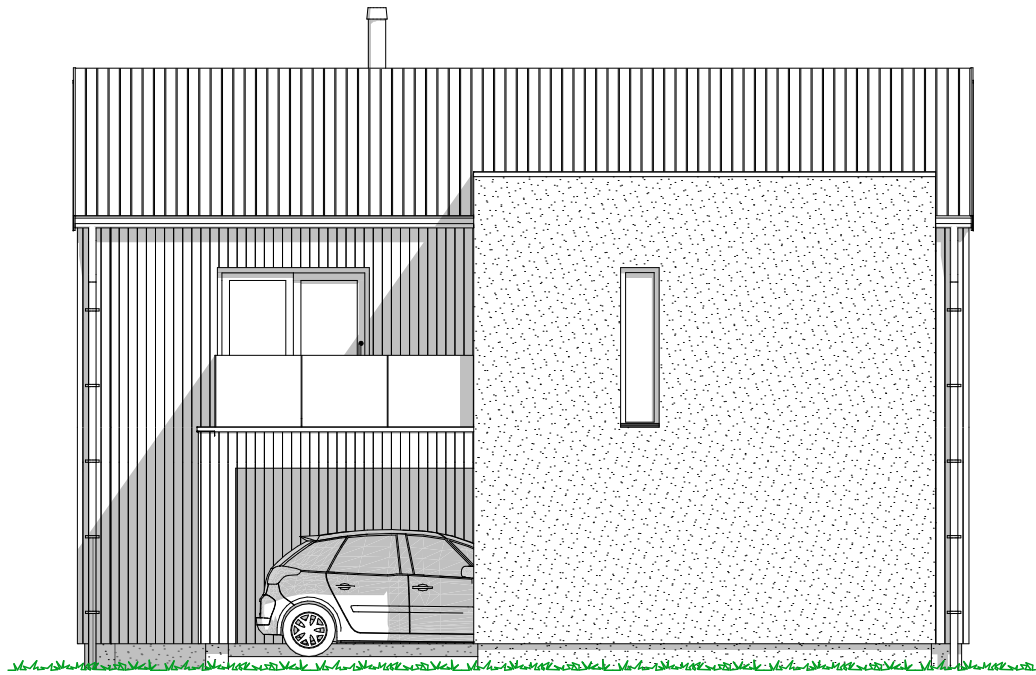
1:100 Fasade Øst
