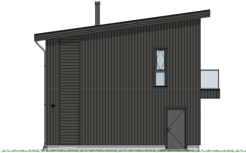
1:100 Fasade Øst
