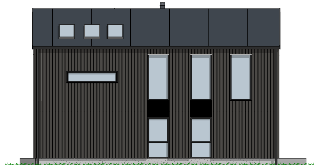
1:100 Fasade Nord
