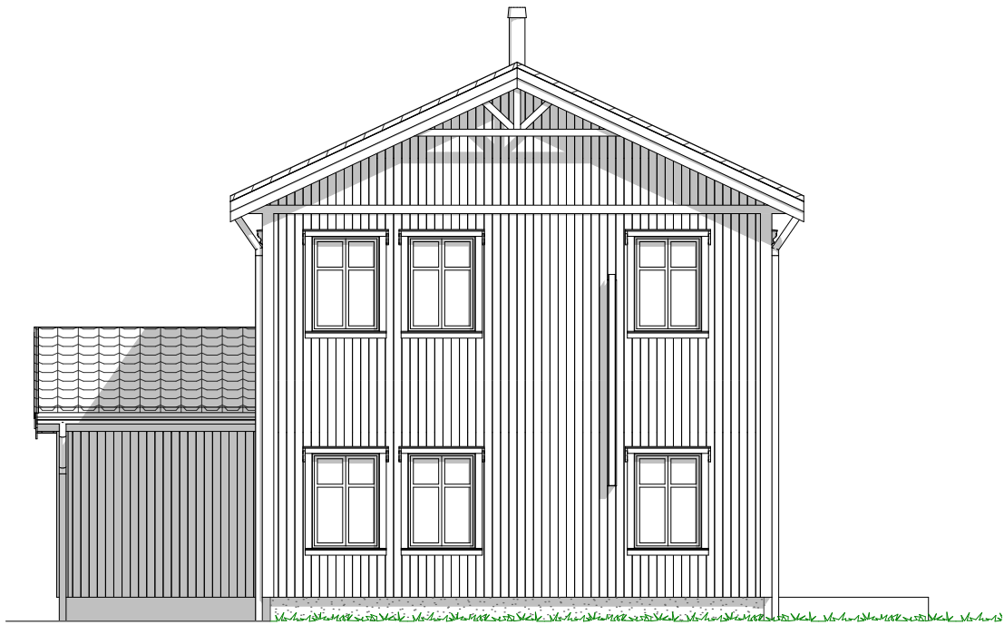
1:100 Fasade NordVest
