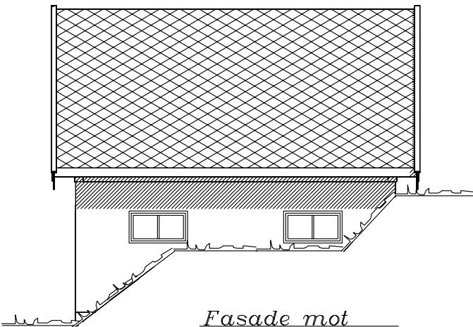
Fasade mot
