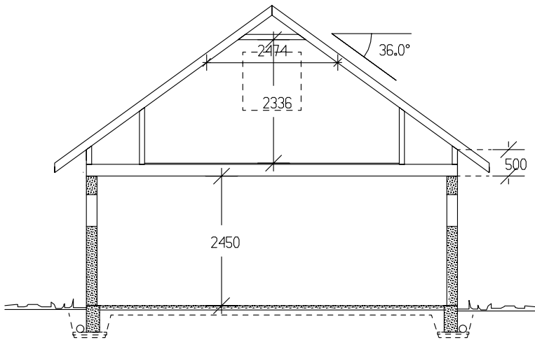
SNITT
