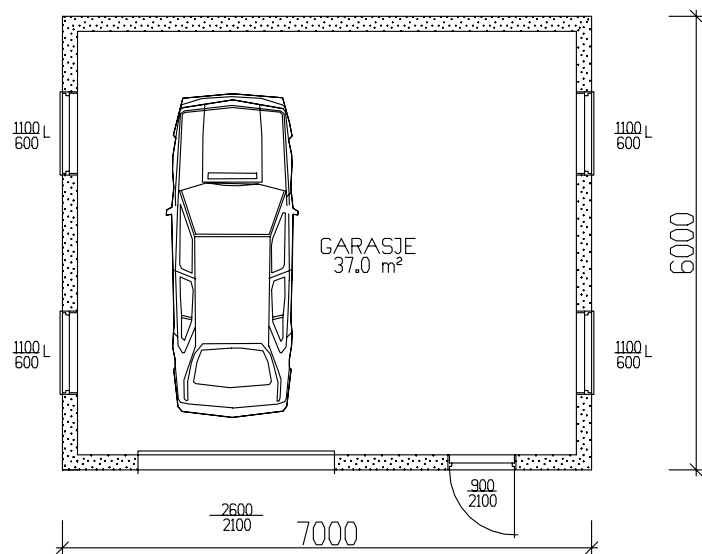
GARASJE 37,0m²BRA
