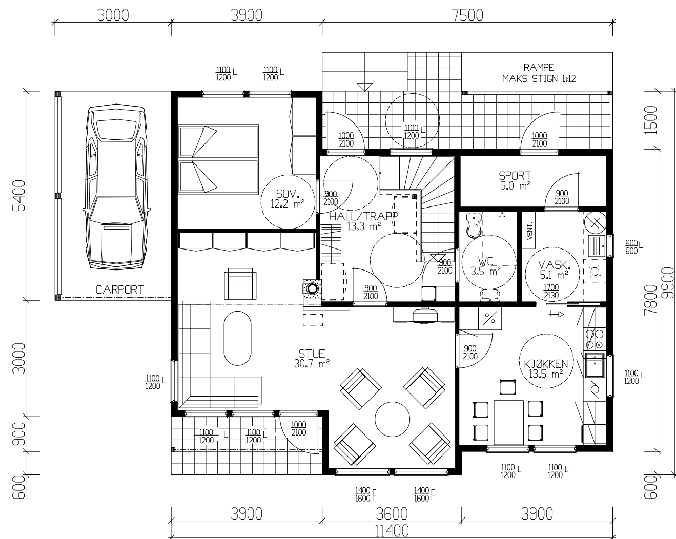
HOVEDPLAN 81.7m 2 BRA-K.+ SPORT 5.0m 2 BRA.
