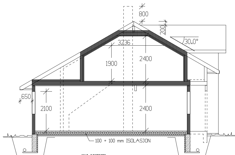
SNITT
