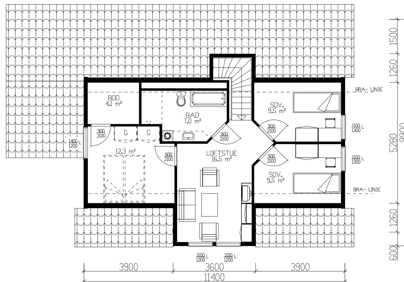
ETASJEPLAN 56,1m 2 BRA-K.
