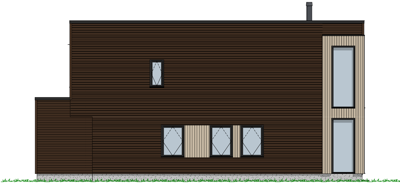
1:100 Fasade Øst
