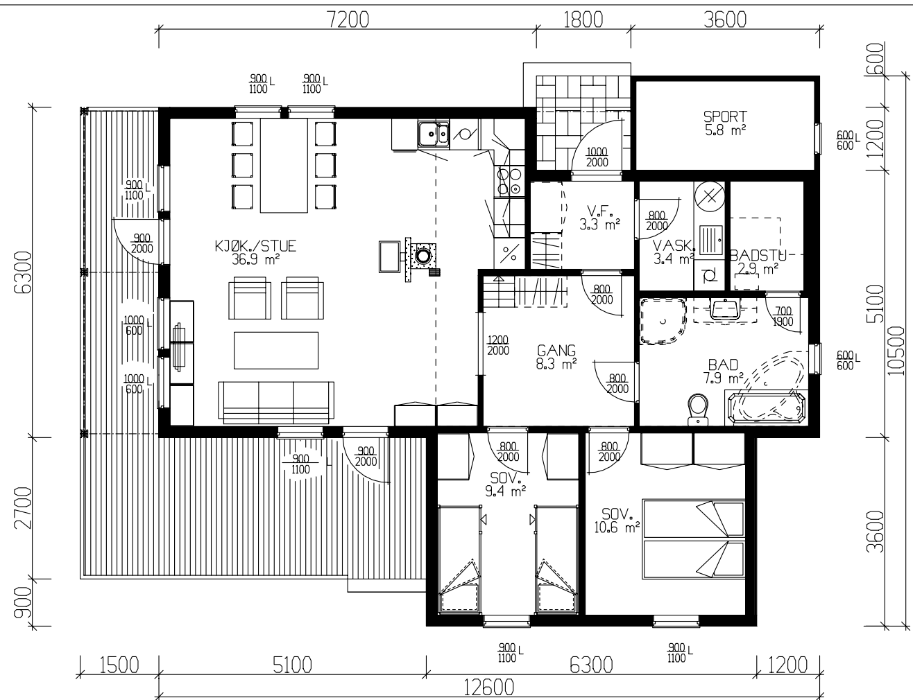
HOVEDPLAN 86,3m² BRA + SPORT 5,8m² BRA
