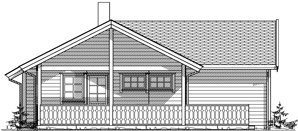
Fasade mot
