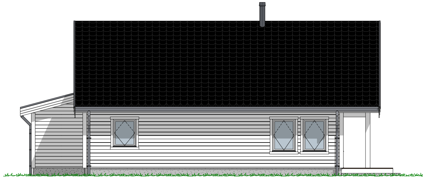
1:100 Fasade Vest Sør Vest
