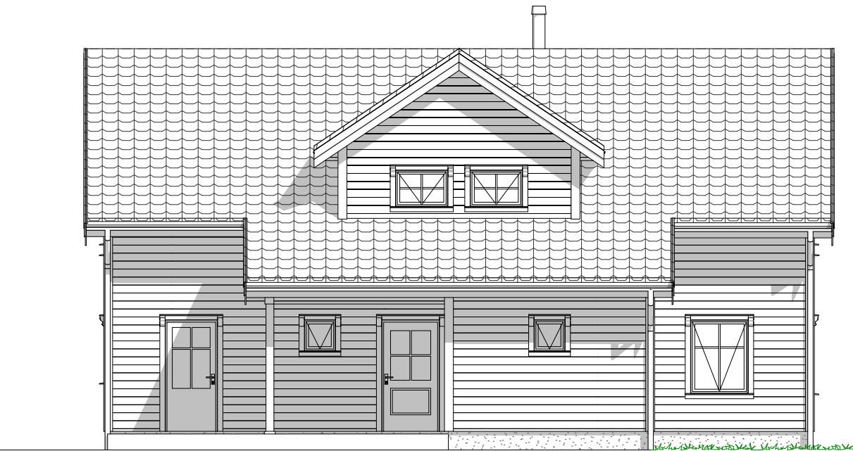
1:100 Fasade Sør-Øst
