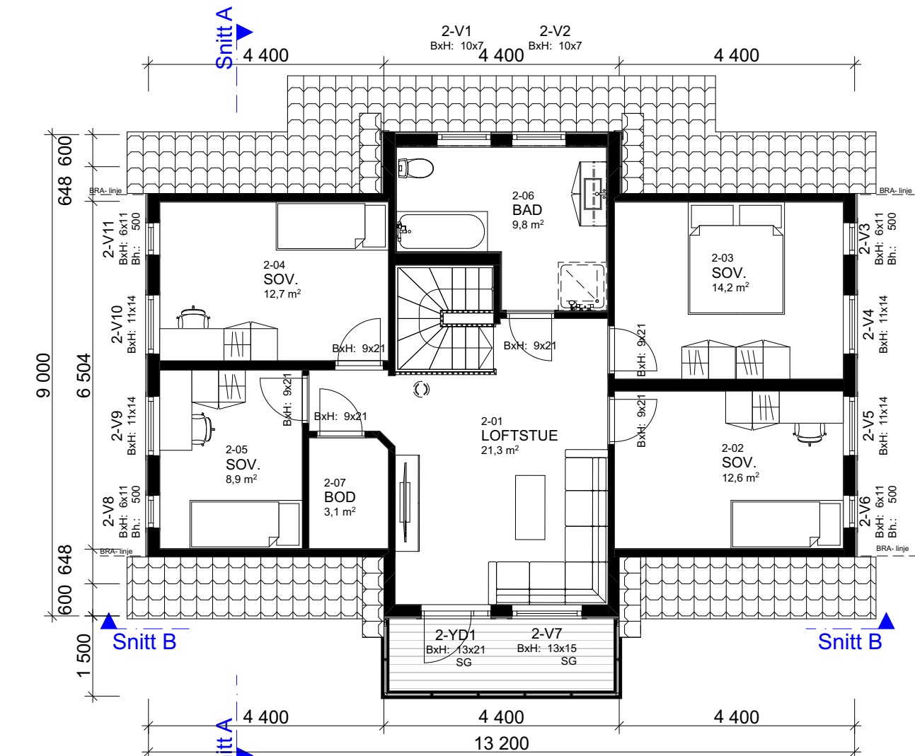
1:100 2. Etasje
