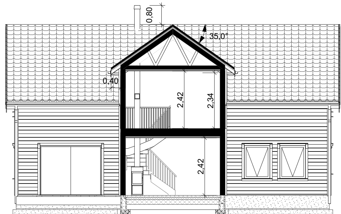
1:100 Snitt B
