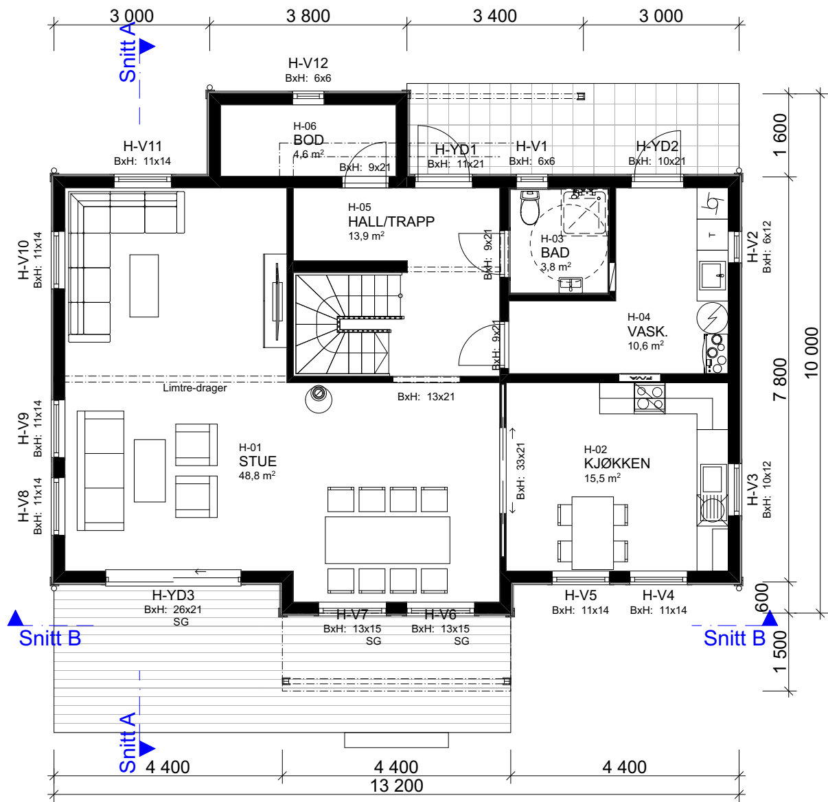
1:100 H. Etasje
