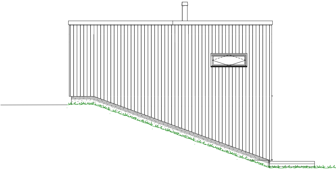
1:100 Fasade sør-øst
