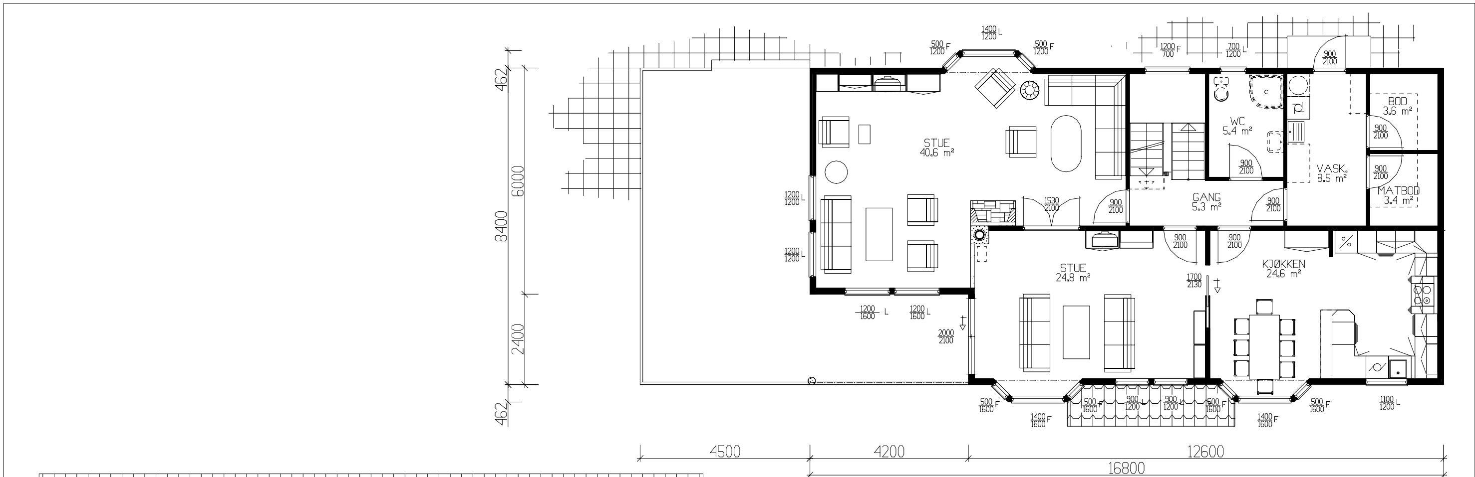
HOVEDPLAN 126.7 m² BRA
