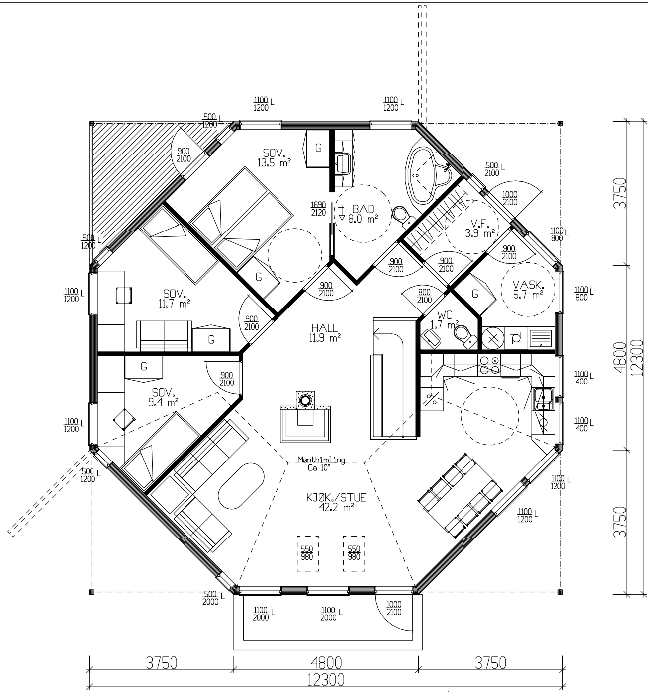
HOVEDPLAN 114,9 m² BRA
