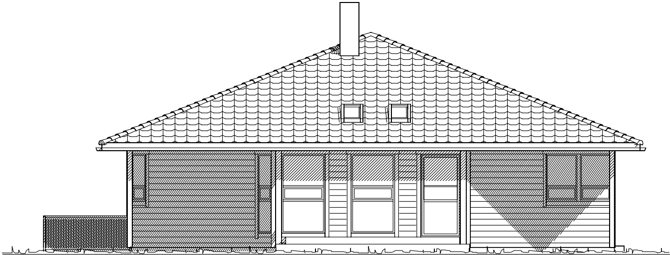
Fasade mot
