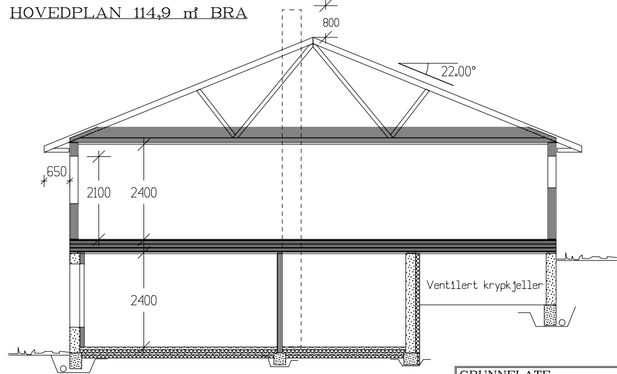
SNITT
