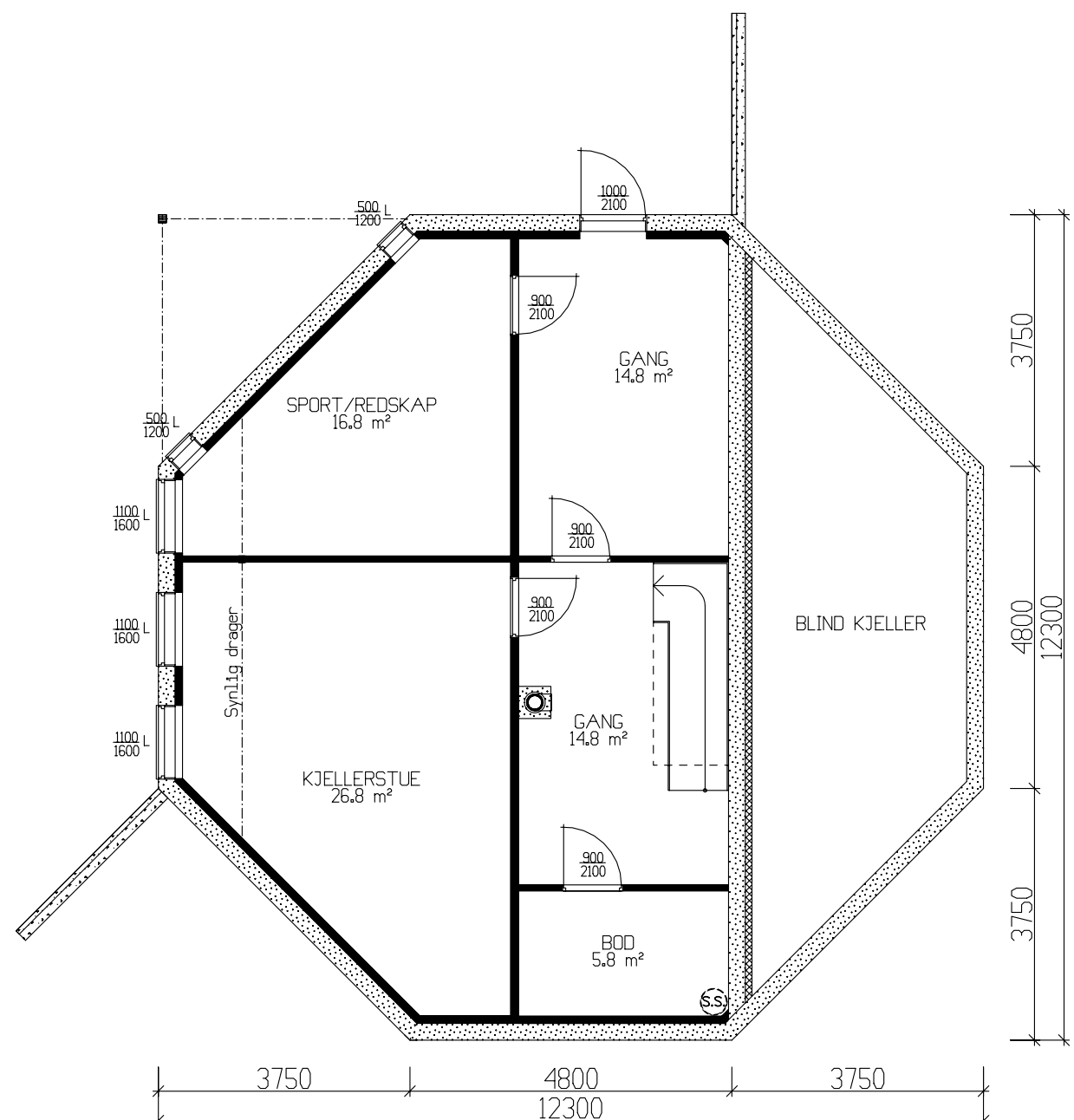
UNDERETASJE 81,7 m² BRA
