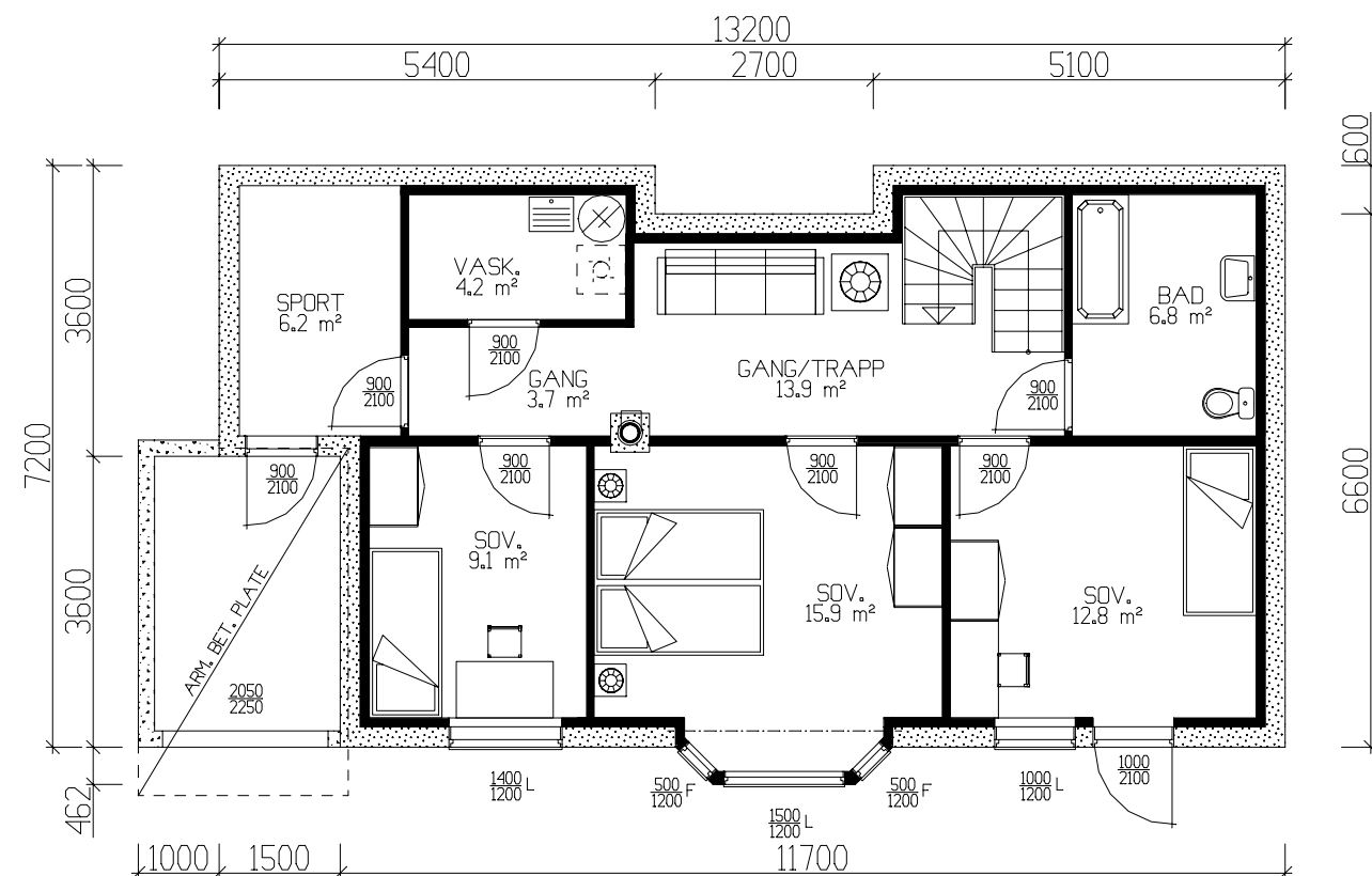
UNDERETASJE 69.5m² BRA-K + SPORT 6.2m² BRA.
