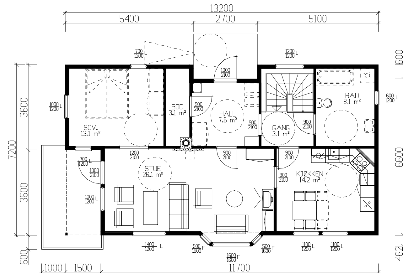
HOVEDPLAN 82.4 m² BRA-K
