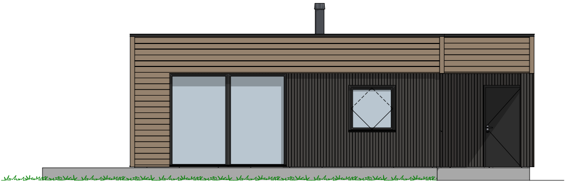
1:100 Fasade Sør
