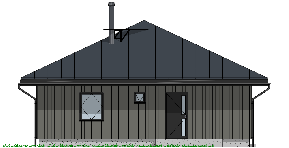
1:100 Fasade Nord Øst
