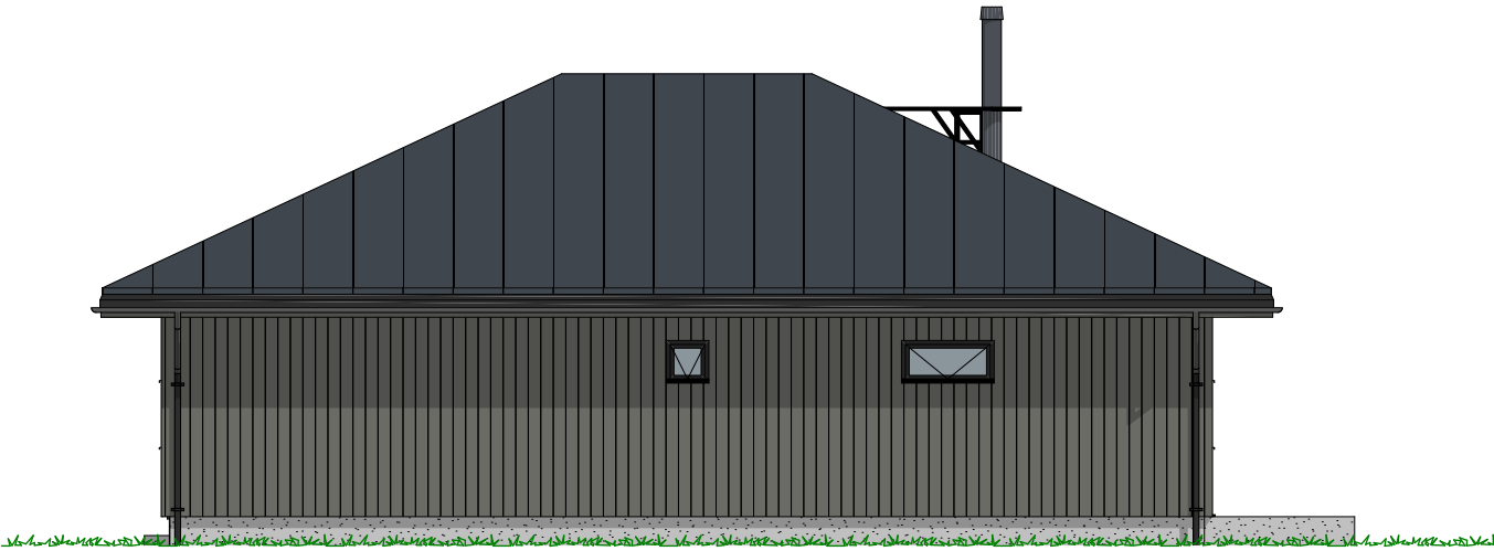
1:100 Fasade Sør Øst
