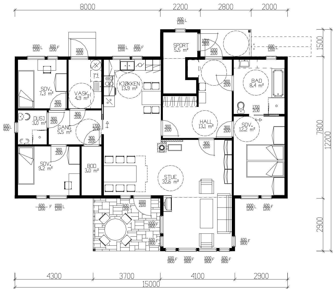
HOVEDPLAN 117,2m² BRA-K + SPORT. 5,5m² BRA
