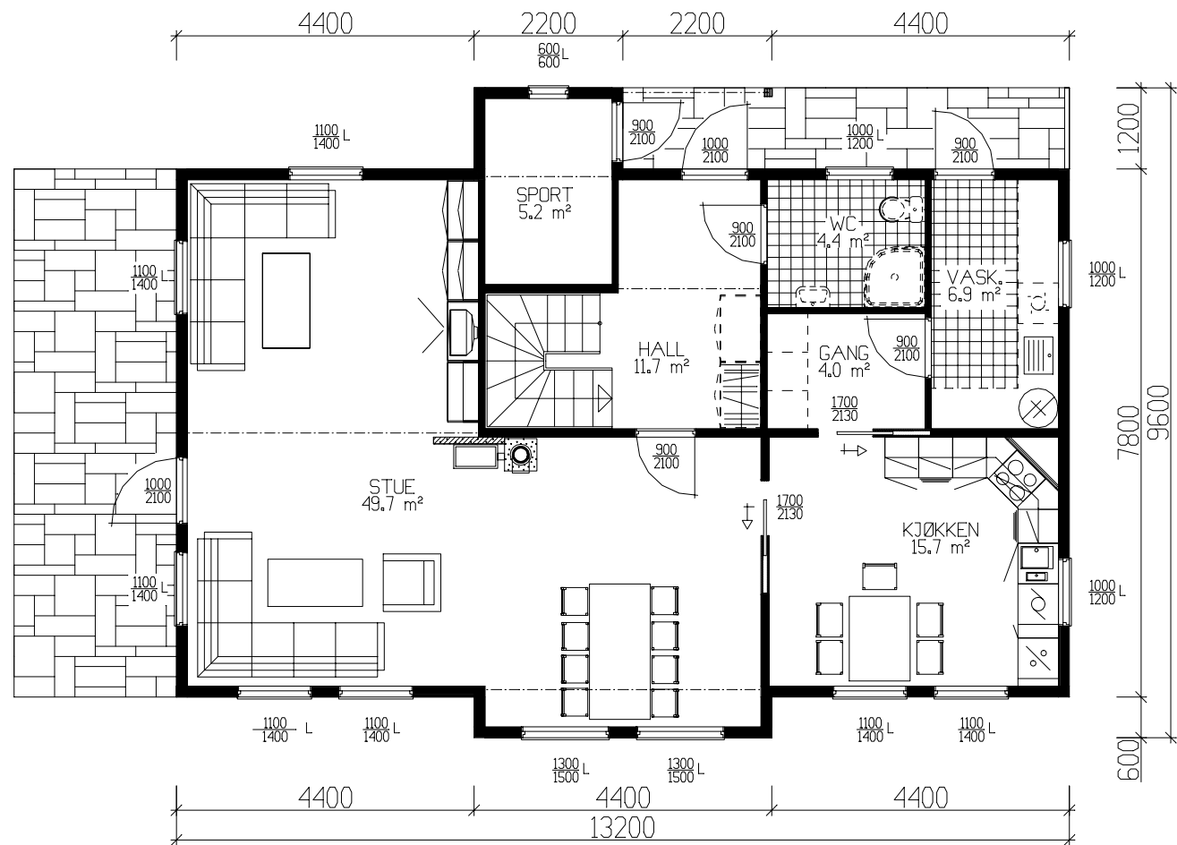
HOVEDPLAN 101.0 m² BRA
