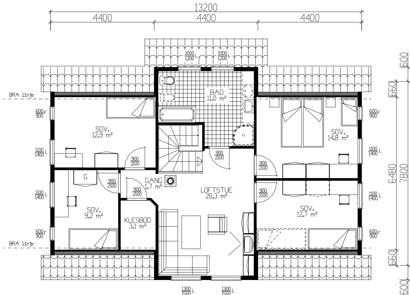
LOFTSPLAN, 91 m² BRA
