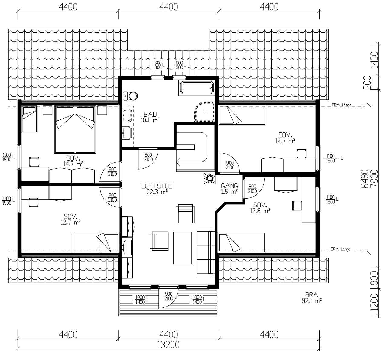
ETASJEPLAN 92.1m² BRA
