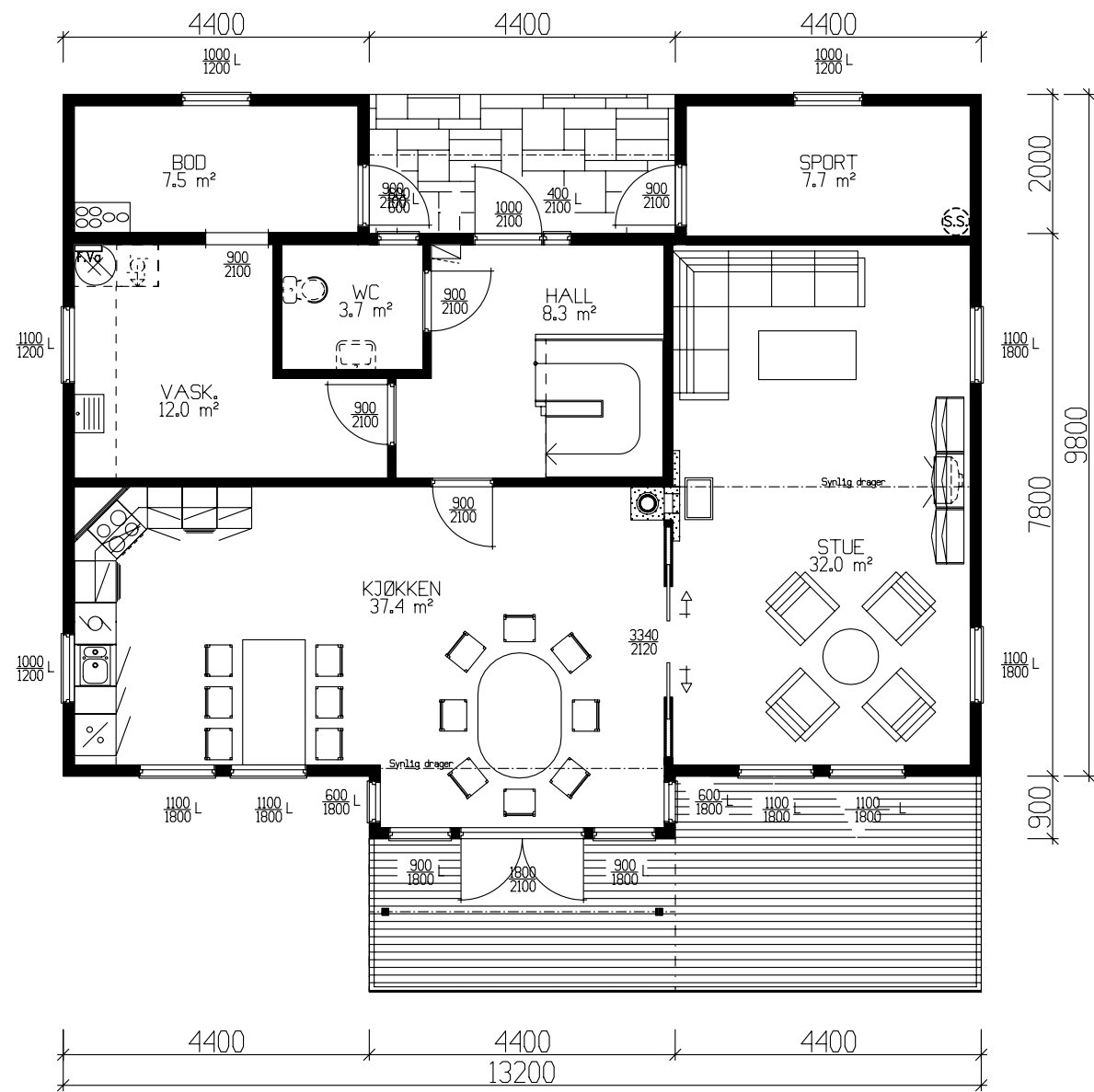
HOVEDPLAN 116.3m² BRA
