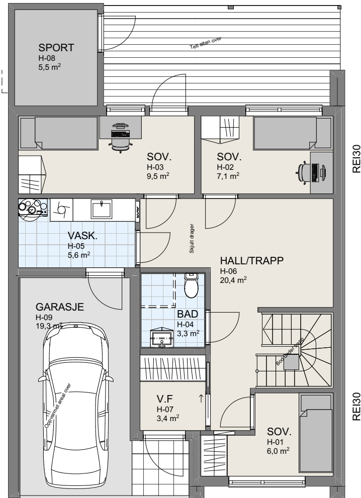
1:100 H. Etasje
