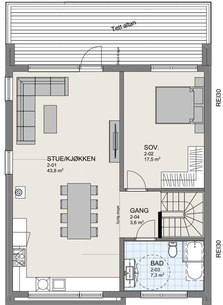
1:100 2. Etasje
