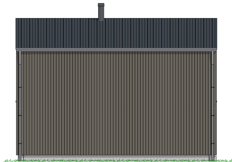
1:100 Fasade Nord
