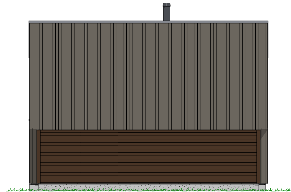
1:100 Fasade Sør
