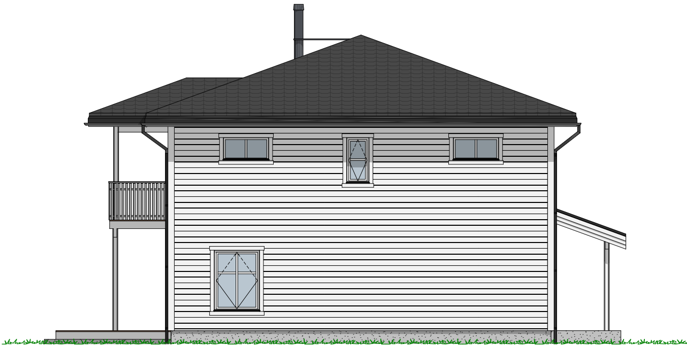
1:100 Fasade Øst
