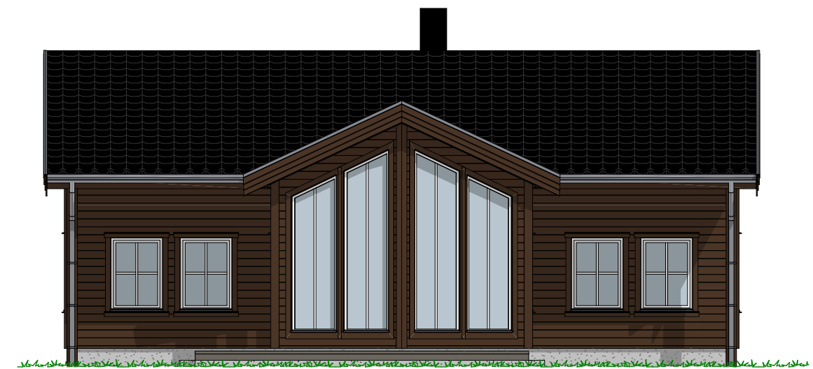
1:100 Fasade Vest
