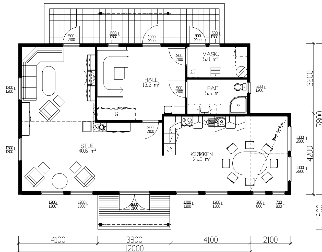
HOVEDPLAN 95.5m² BRA.
