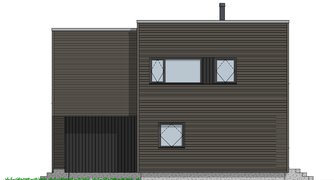
1:100 Fasade Øst
