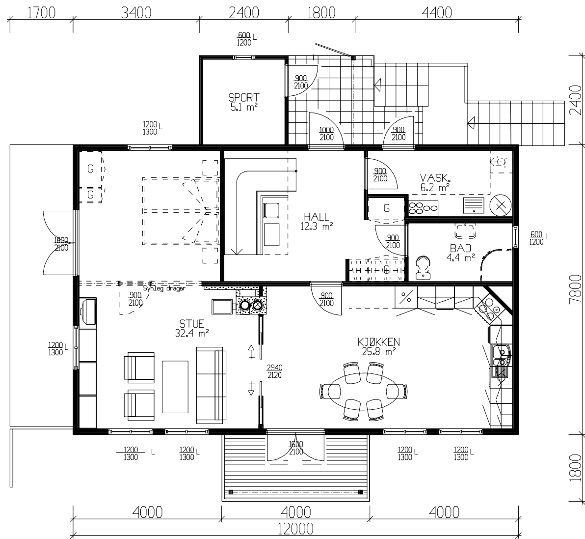
HOVEDPLAN 87.4m² BRA + SPORT 5.1m² BRA
