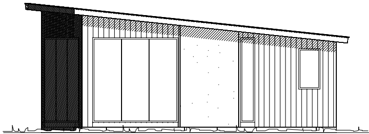
Fasade mot _____
