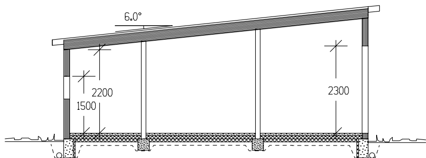
SNITT
