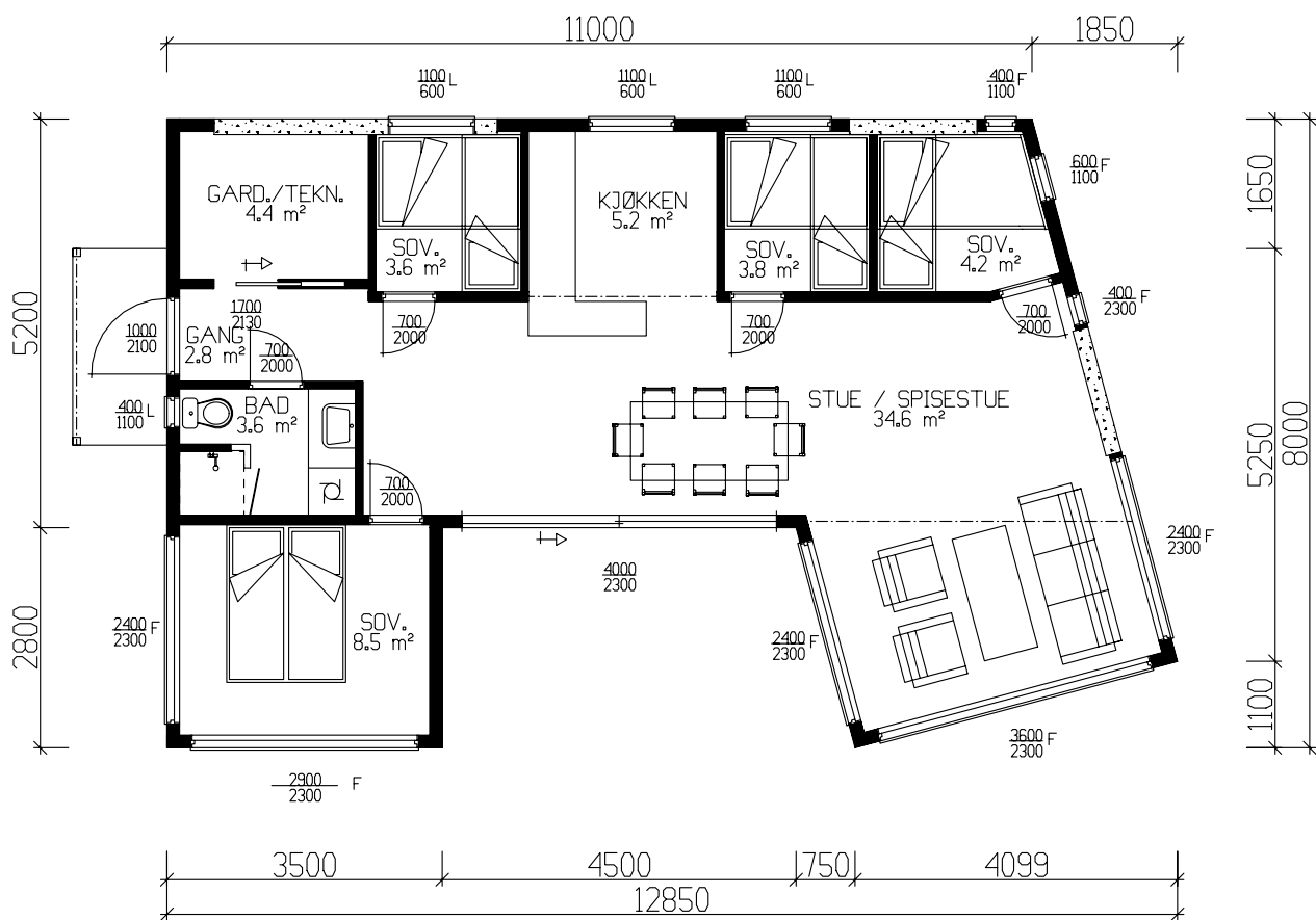
HOVEDPLAN 73,3m² BRA
