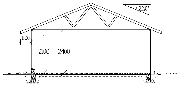
SNITT
