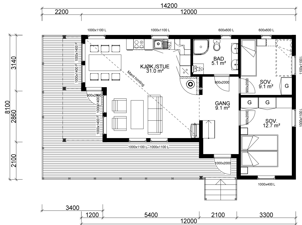
HOVEDPLAN: 69,1 m² BRA
