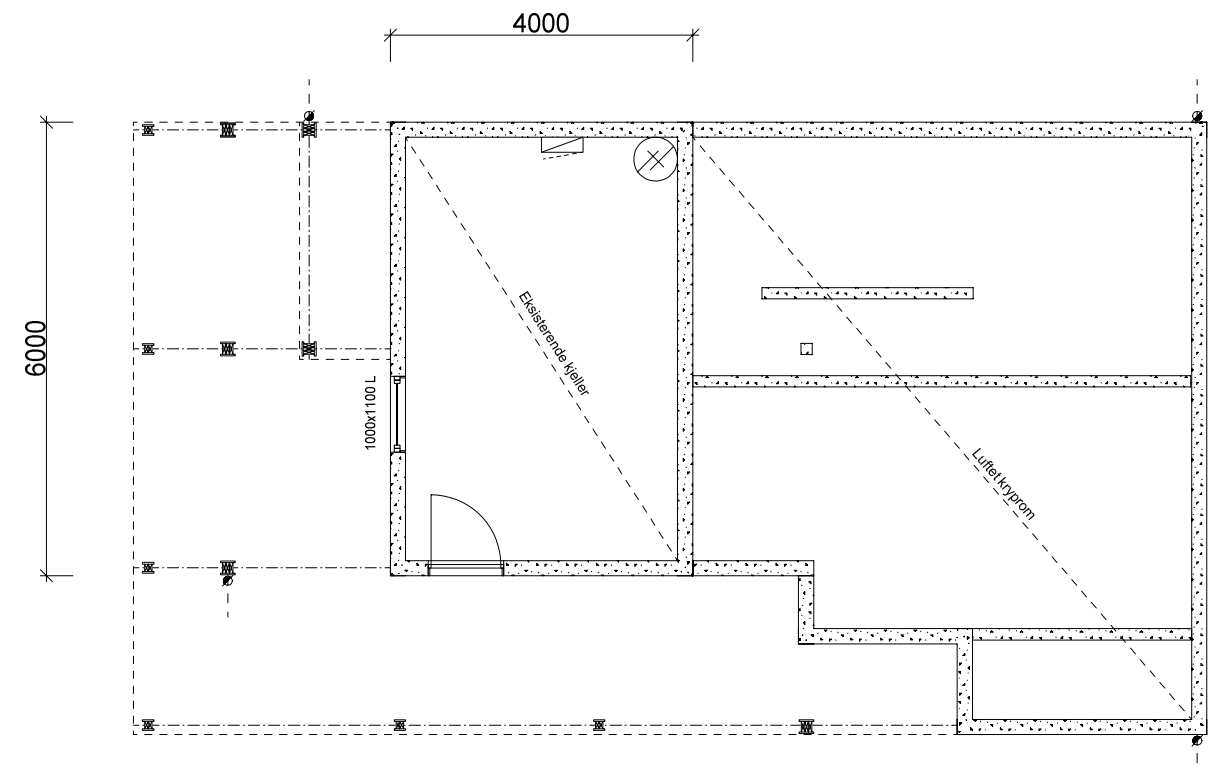
KJELLERPLAN.
