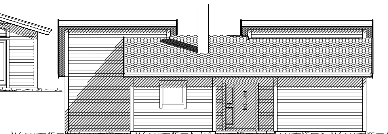
Fasade mot
