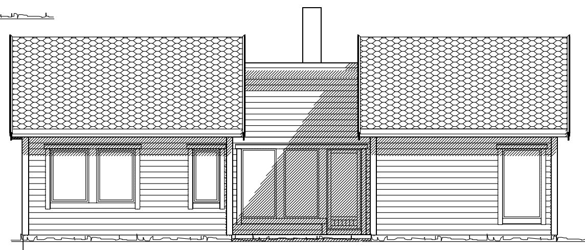
Fasade mot
