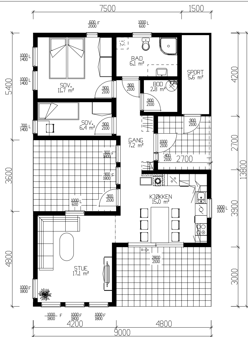
HOVEDPLAN 69.8m² BRA + SPORTSBOD 5.6m²
