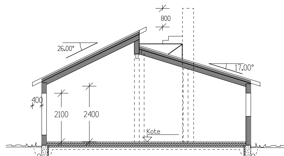
SNITT
