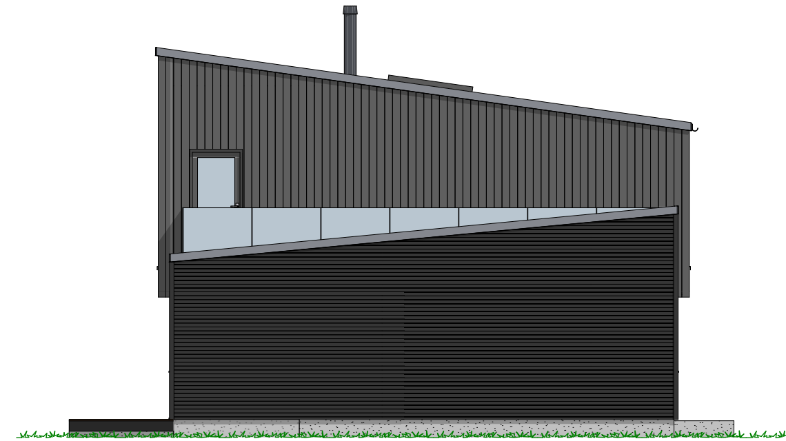
1:100 Fasade Sør
