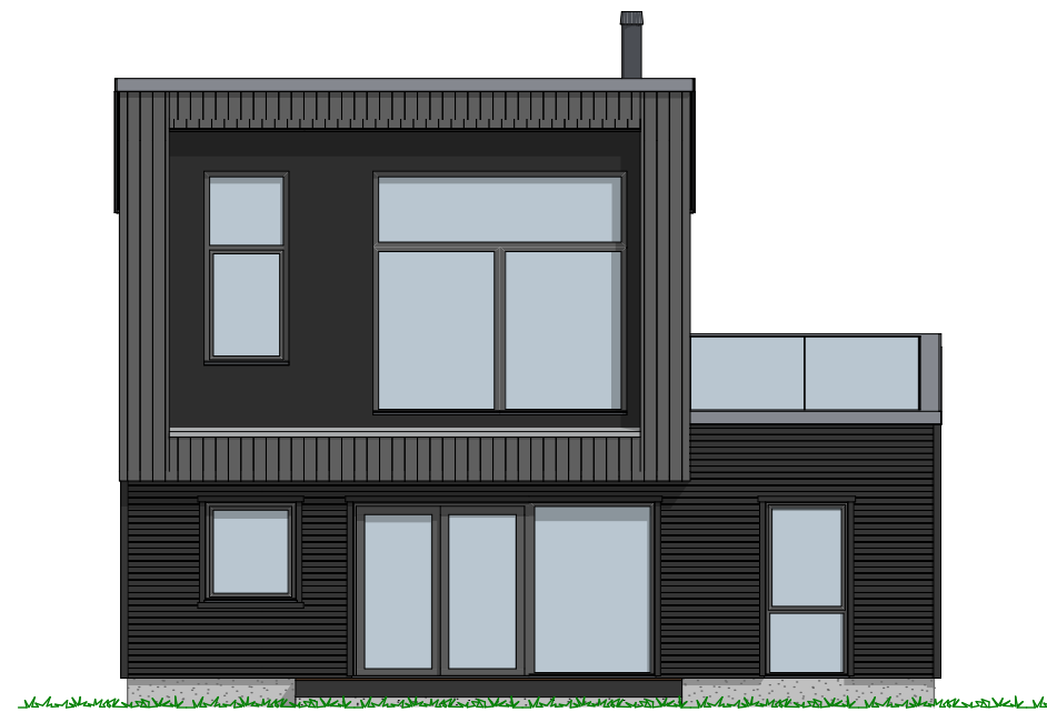
1:100 Fasade Vest
