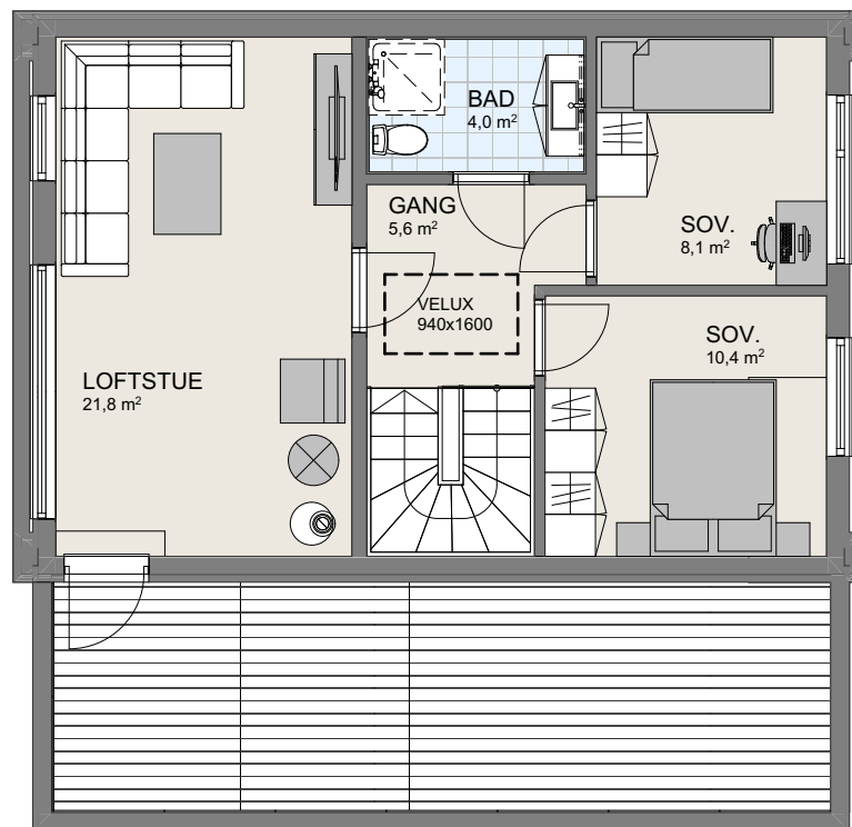
1:100 2.Etasje
