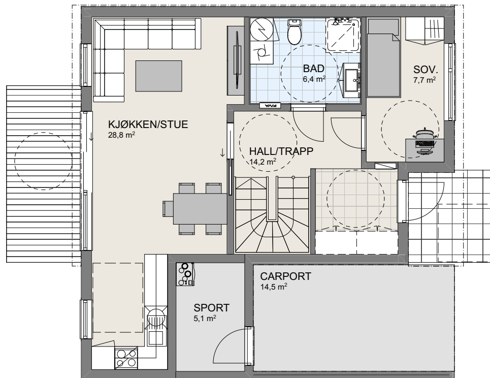
1:100 H. Etasje
