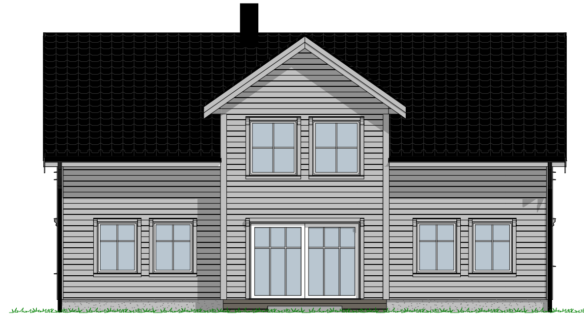
1:100 Fasade Nord Vest
