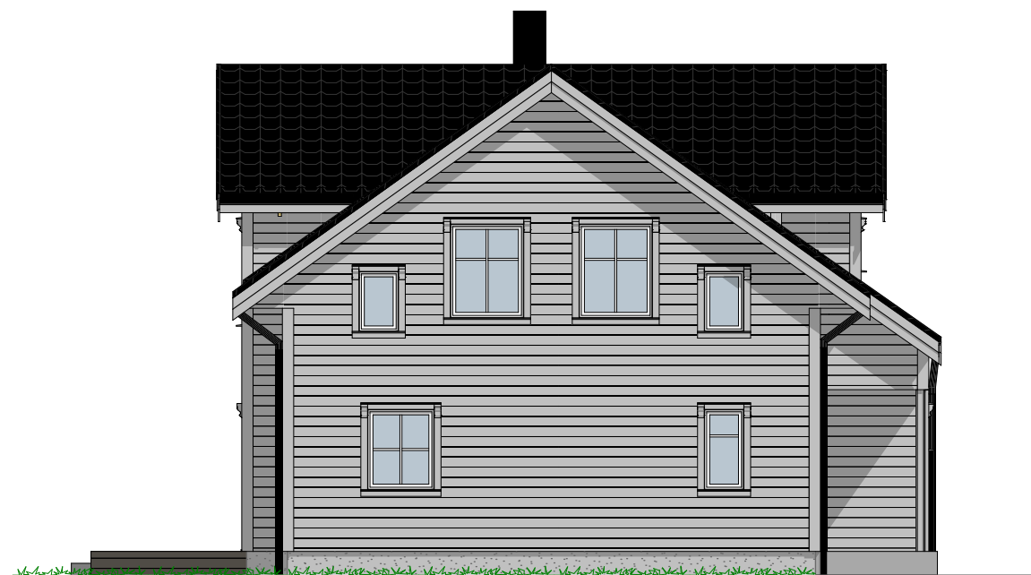
1:100 Fasade Sør Vest
