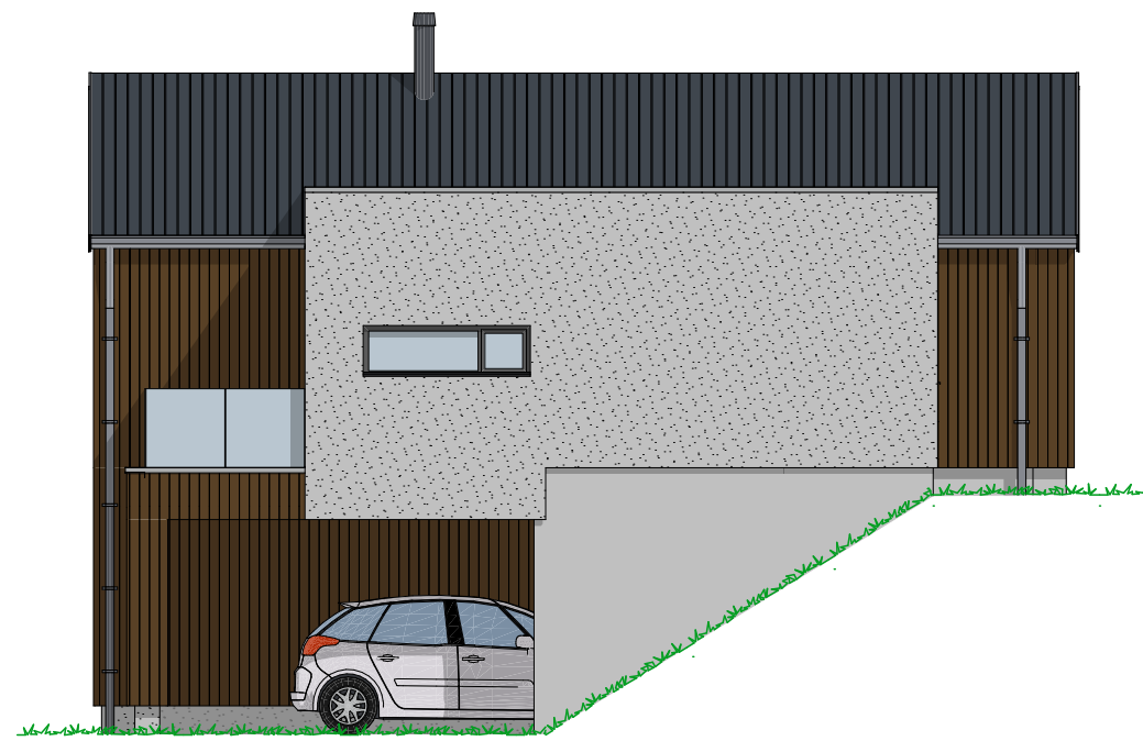
1:100 Fasade Øst
