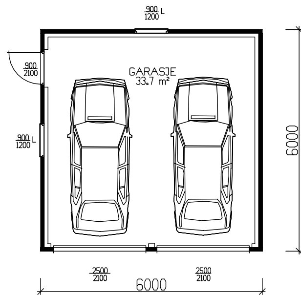
GARASJE 33,7m² BRA
