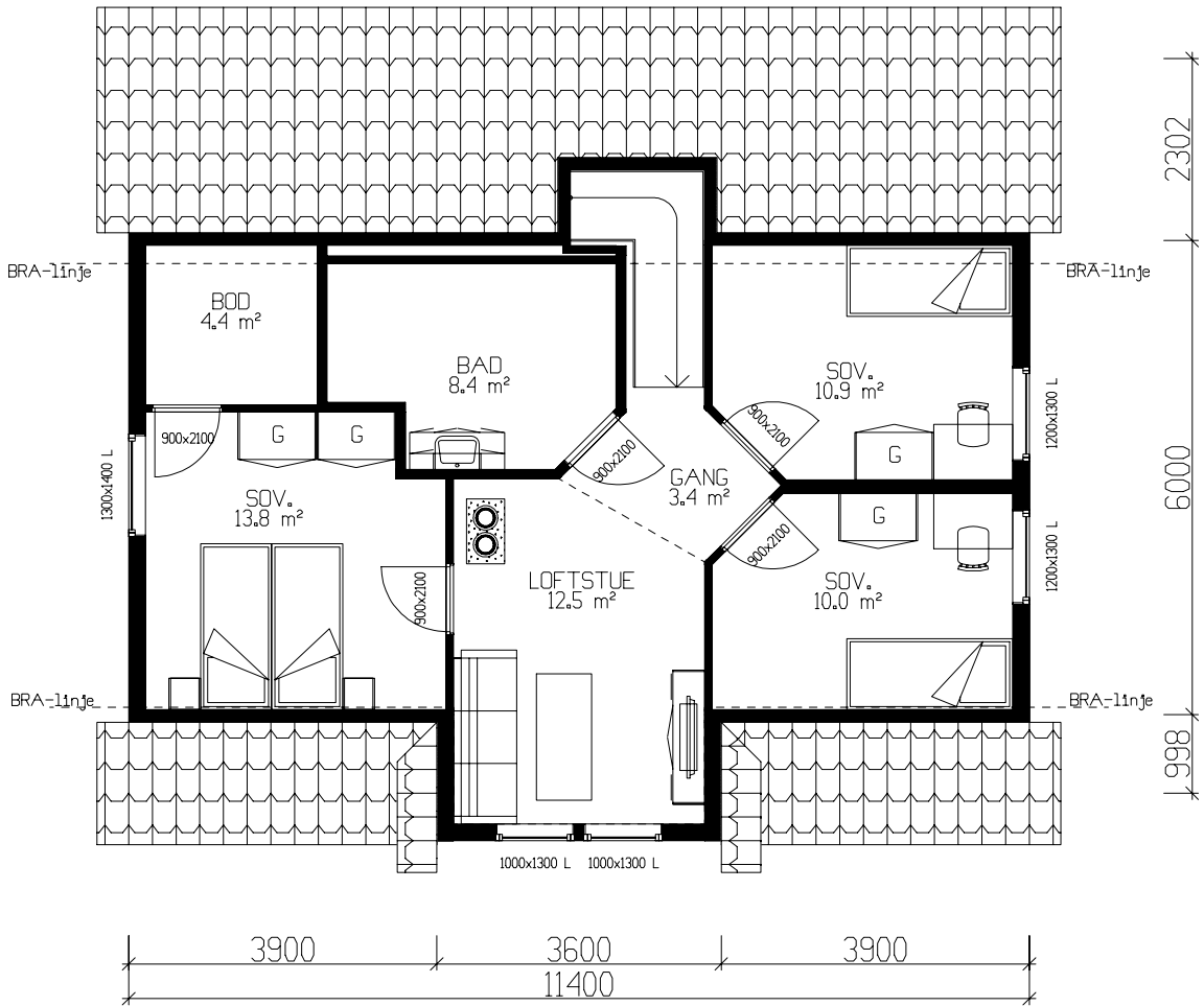
ETASJEPLAN LOFT: 66,4m² BRA
