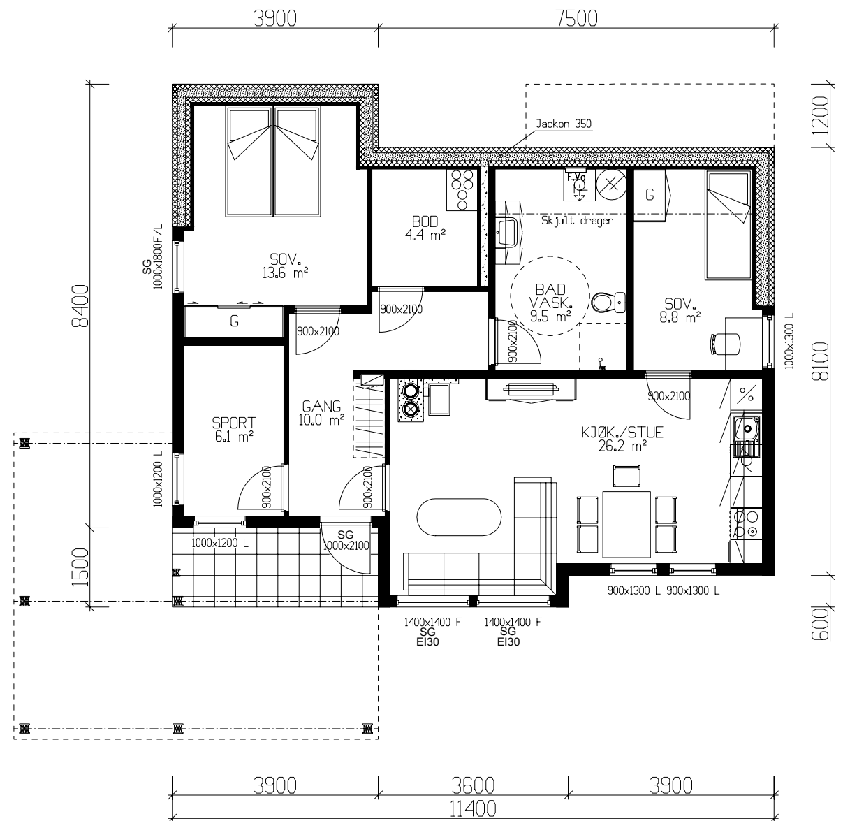
UNDERETASJE: 83,2m² BRA
