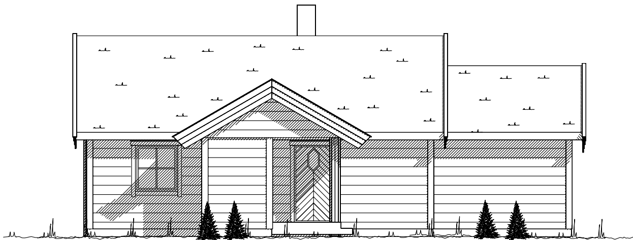
Fasade mot
