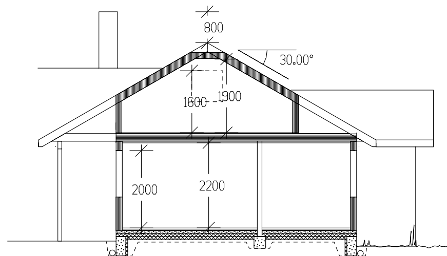
SNITT-HEMS
