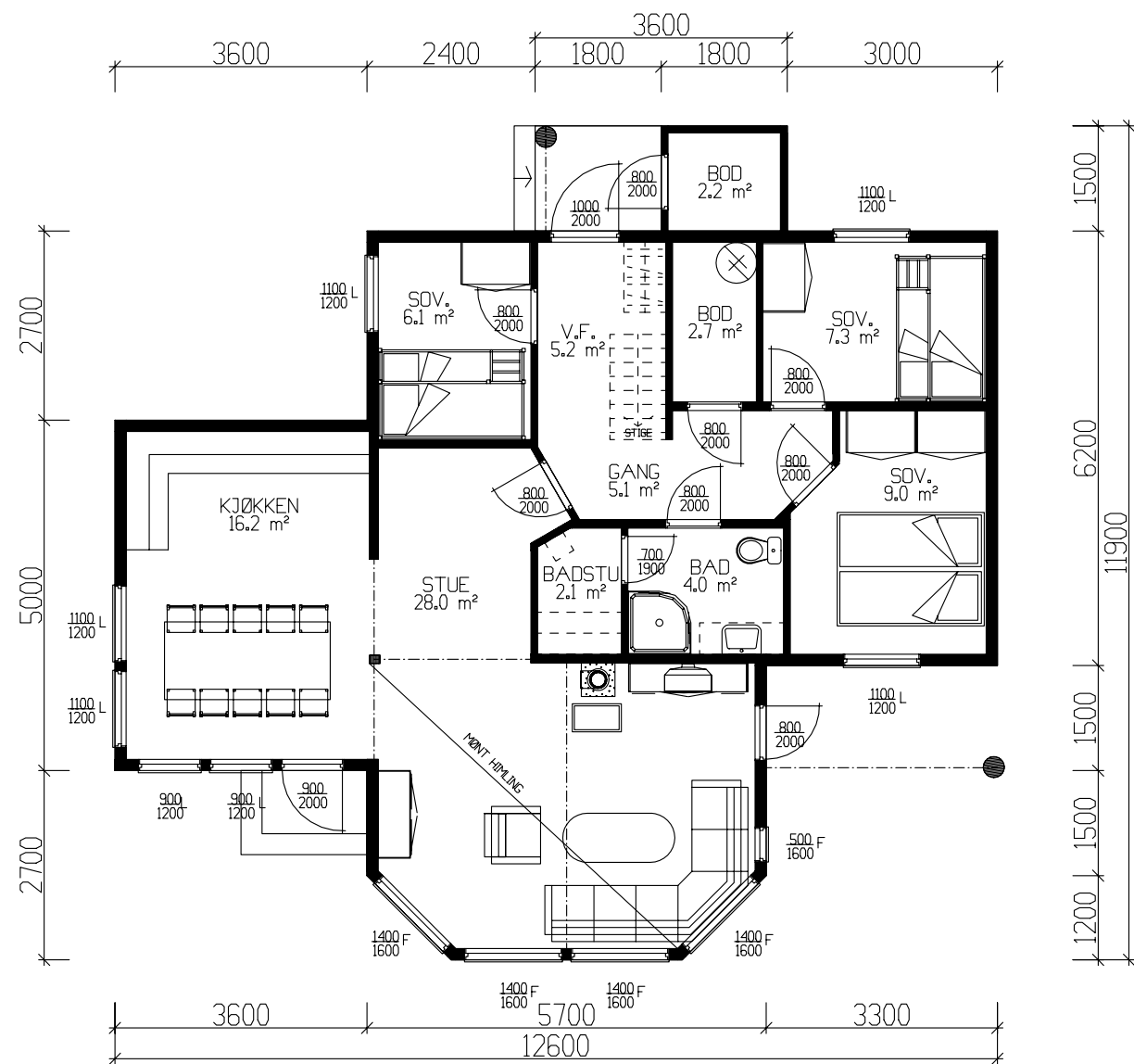
HOVEDPLAN 89,3 m² BRA
