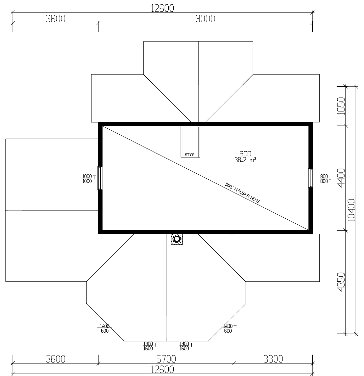
IKKE MALBAR BOD 38,2 m²
