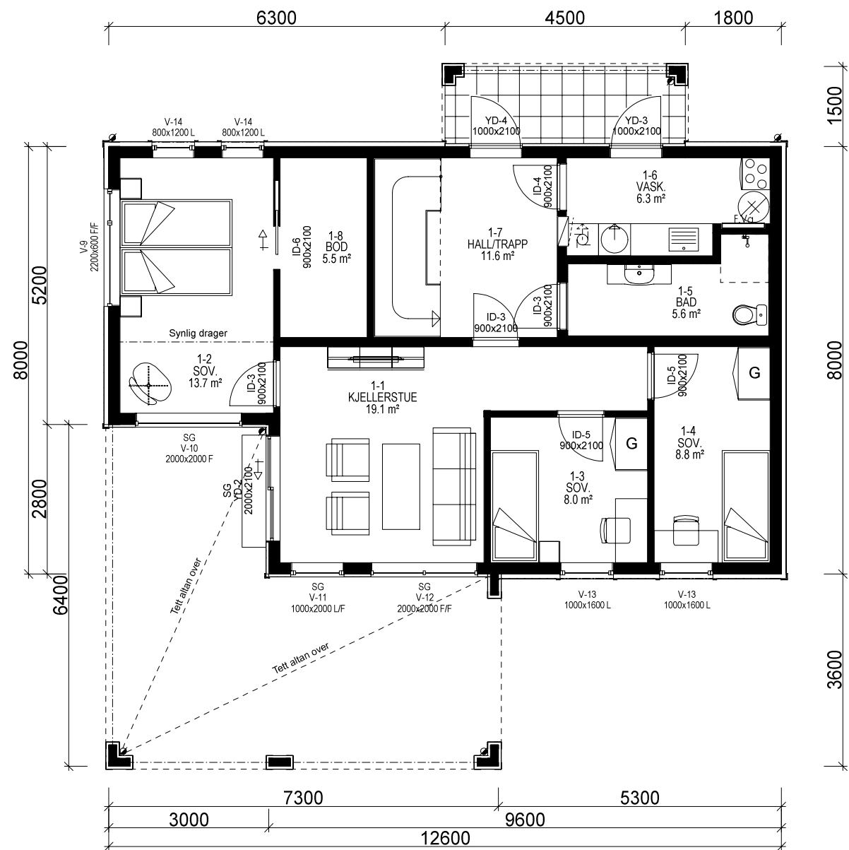
H. ETG. PLAN 1: 83,9 m² BRA
