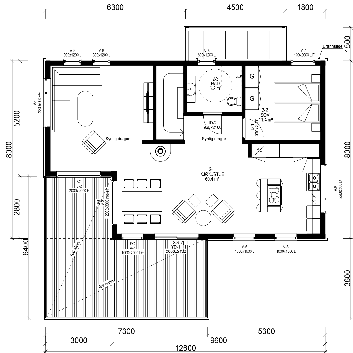
H. ETG. PLAN 2: 83,9 m² BRA
