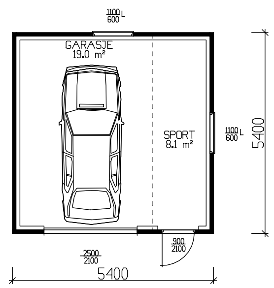
GARASJE 27,1m² BRA
