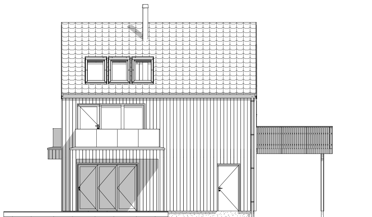
1:100 Fasade Vest
