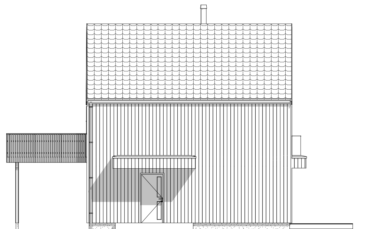
1:100 Fasade Øst
