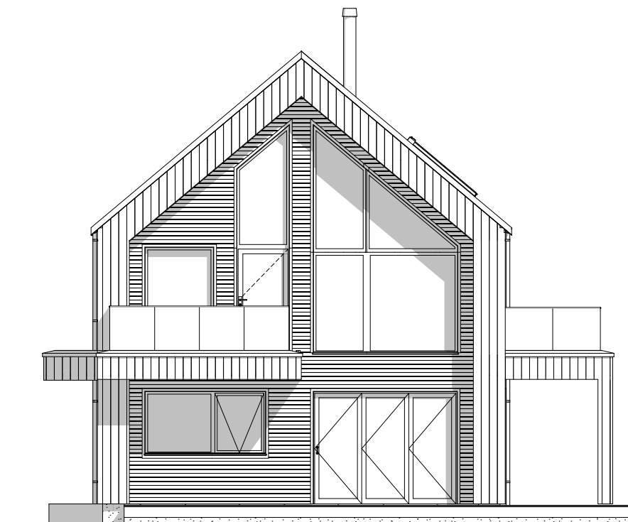
1:100 Fassade Nord
