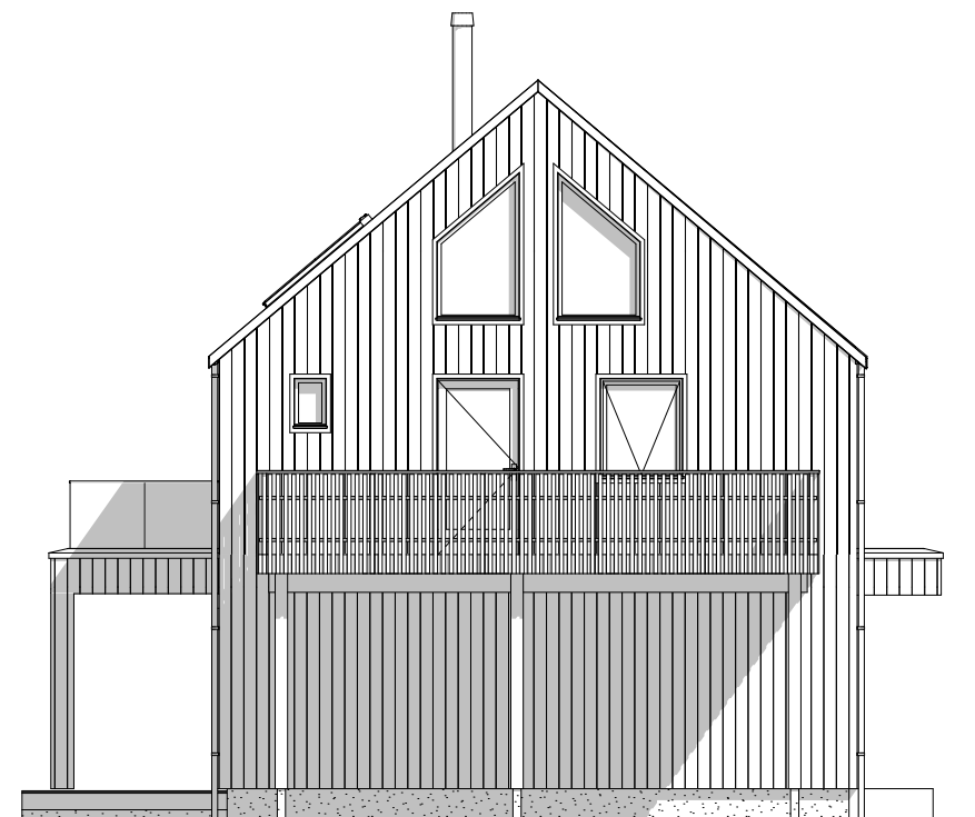
1:100 Fasade Sør
