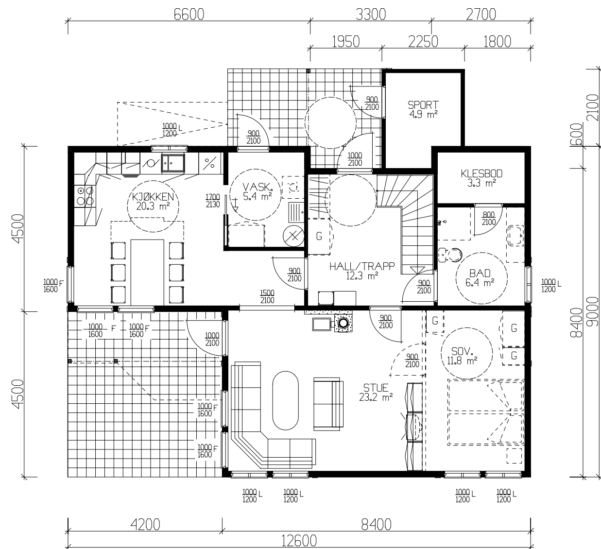
HOVEDPLAN 85.5m² BRA-K. SPORT 5.0m² BRA.
