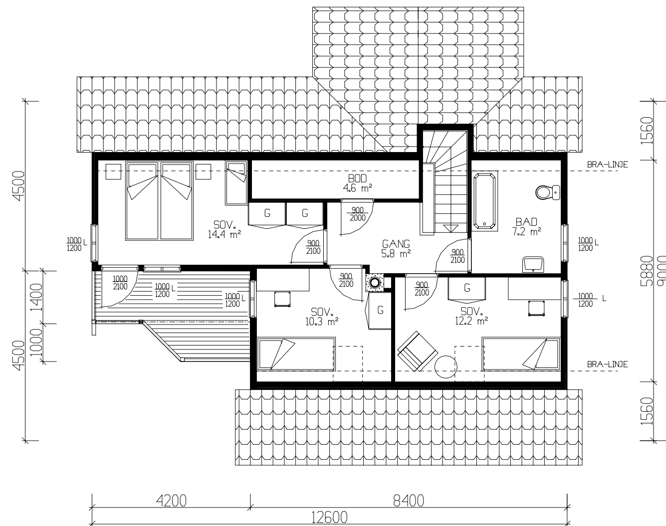
ETASJEPLAN LOFT 53.3m² BRA-K.
