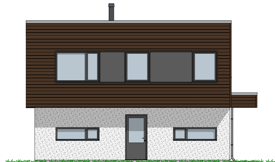
1:100 Fasade Sør
