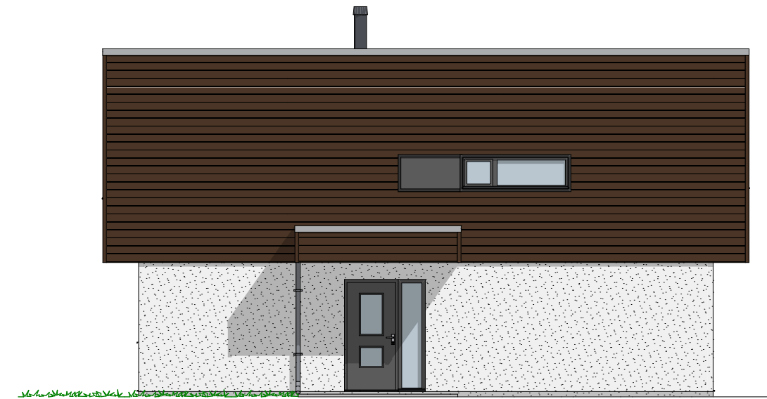
1:100 Fasade Øst
