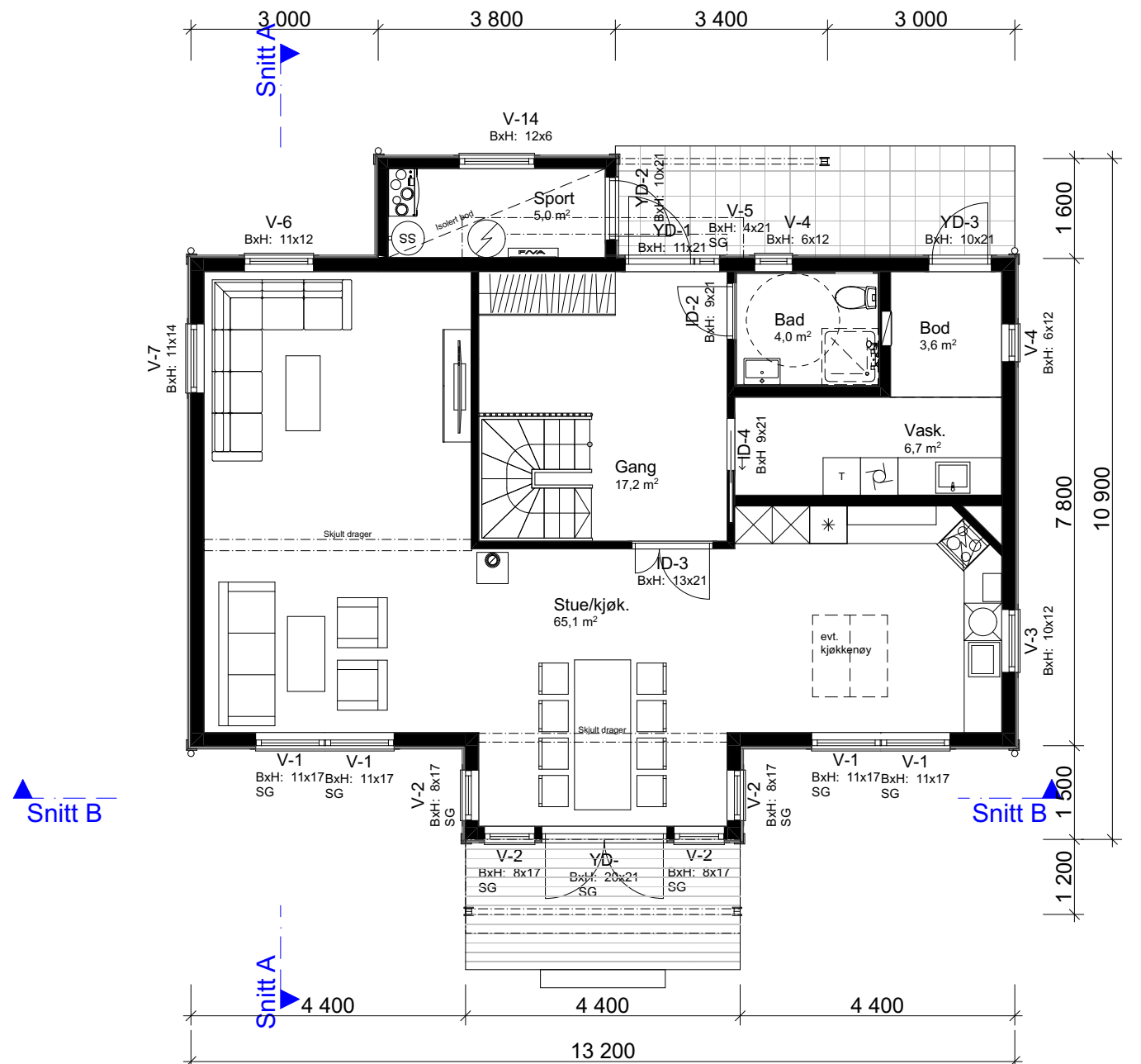
1:100 H. Etasje
