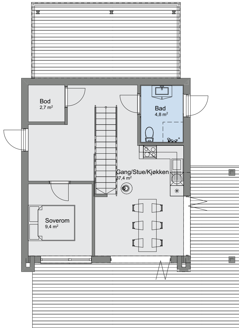
1:100 H. etasje
