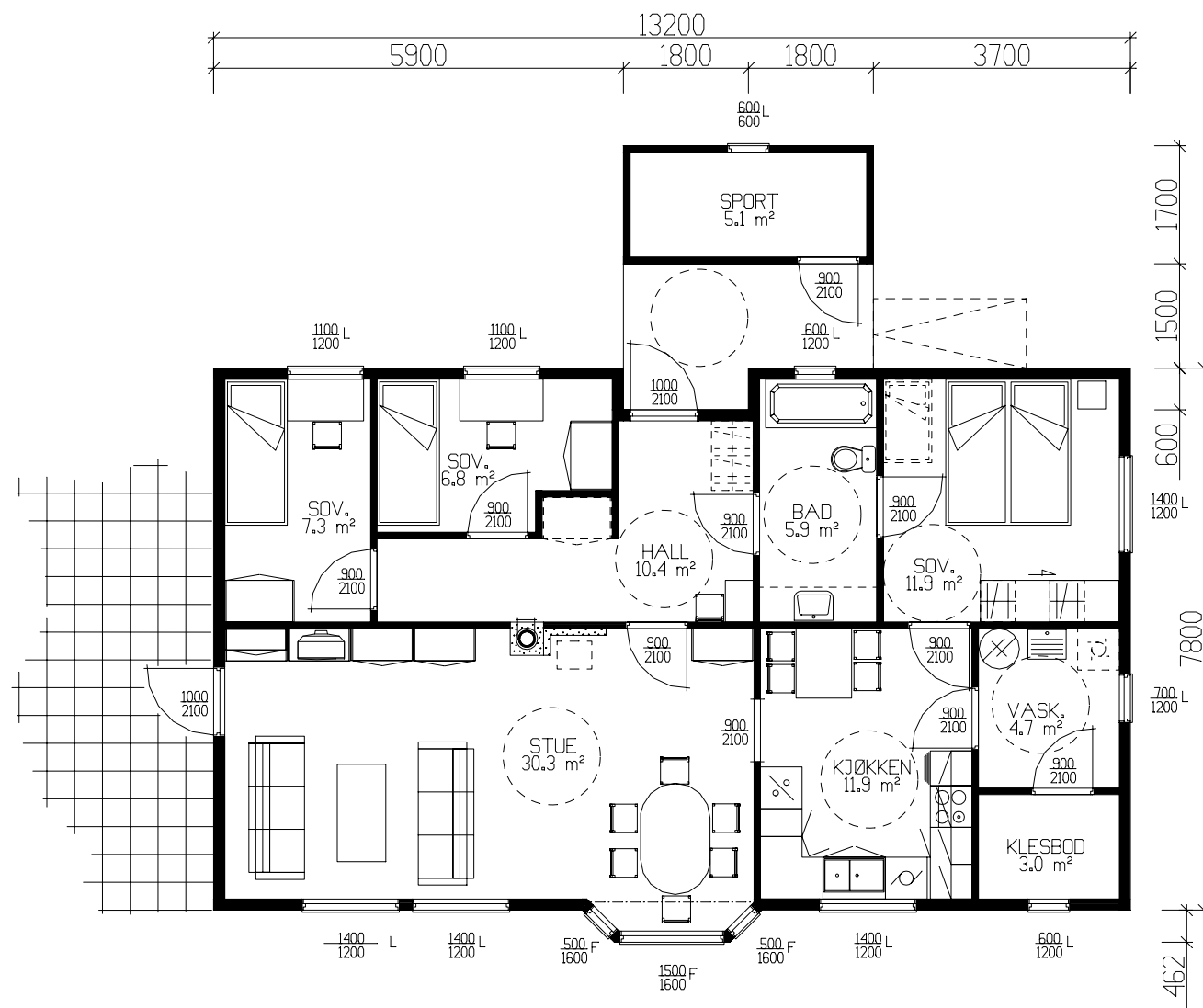
HOVEDPLAN 96.0m² BRA-K + SPORT 5.1m² BRA.
