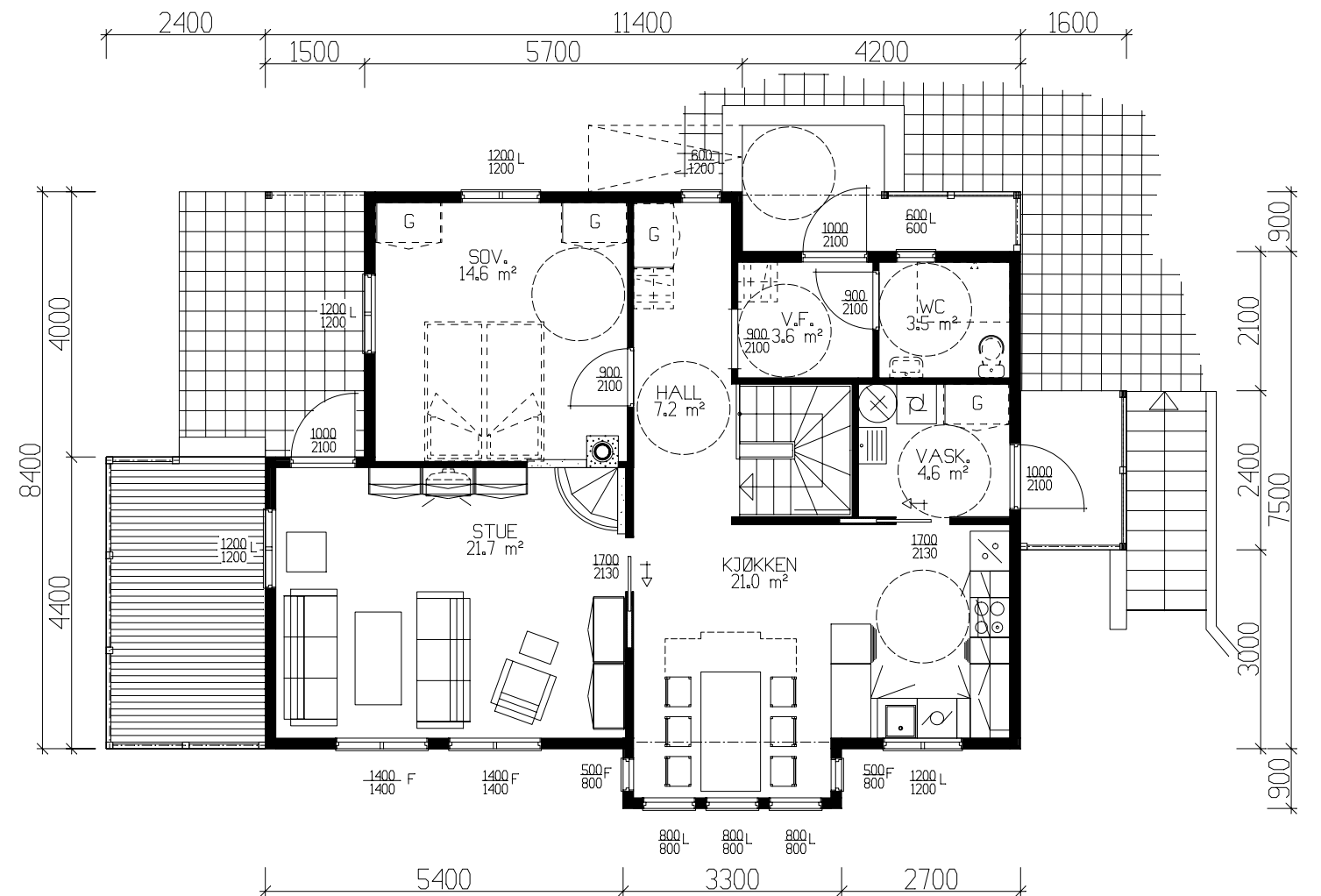
HOVEDPLAN 82.4 m² BRA
