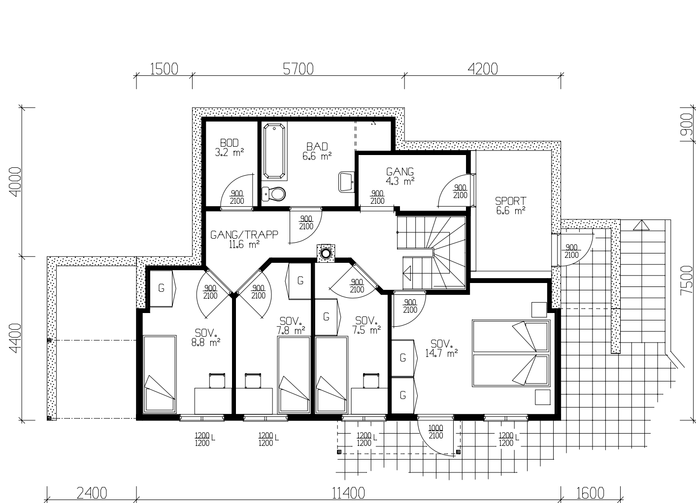
UNDERETASJE 69.5 m² BRA-K + sport 6.6 m² BRA.
